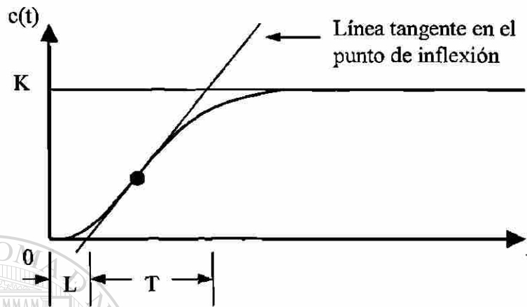
Figura 4.1: Curva de respuesta con forma de "S".
