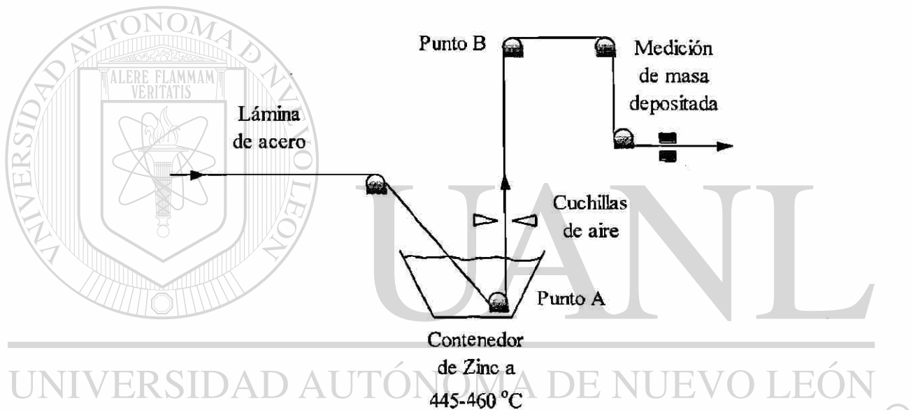
Figura 1.1: Proceso de galvanización.
