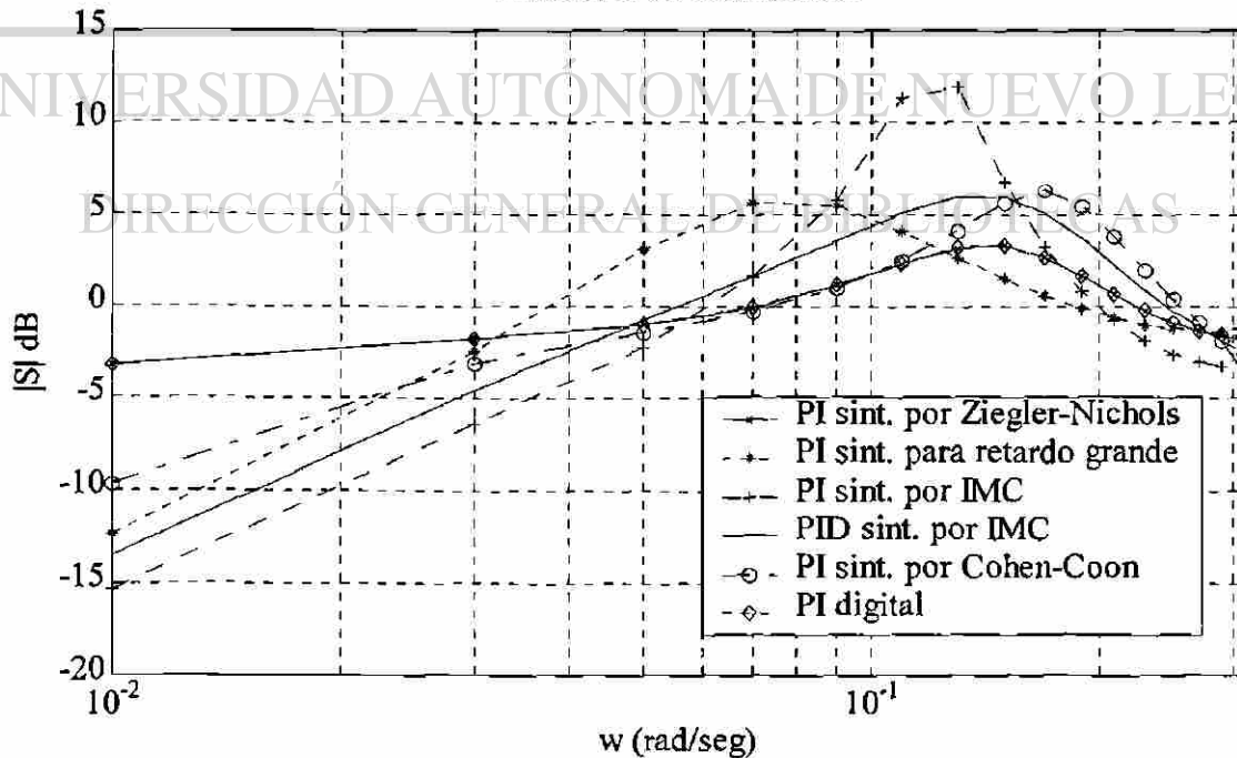
Funciones de sensibilidad
