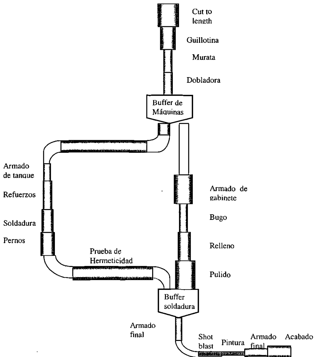
Figura 3.3.1.1. Representación de la capacidad de la planta en forma de Tubería
