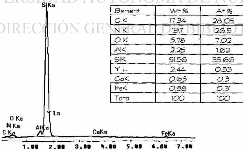
Fig. 5.42 EDS general de la muestra sinterizada con 2,5% de Y_2O_3 - Al_2O_3 .
