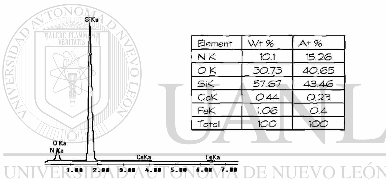
DIRECCIÓN GENERAL DE BIBLIOTECAS Fig. 5.20 EDS de la ceniza pirolizada en atmósfera de nitrógeno a 1250°C por 6 horas.
