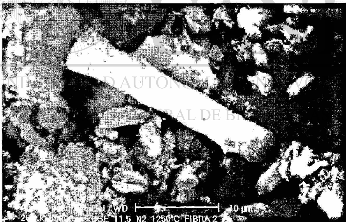
Fig. 5,19 Micrografía de la ceniza pirolizada a 1250°C por 6 hrs. en atmósfera de nitrógeno.
