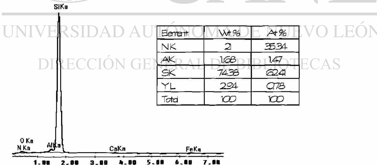
Fig. 5,26 EDS de partículas encontradas en la muestra sinterizada de composición x = 0,5\% de Y_2O_3 - Al_2O_3 .
