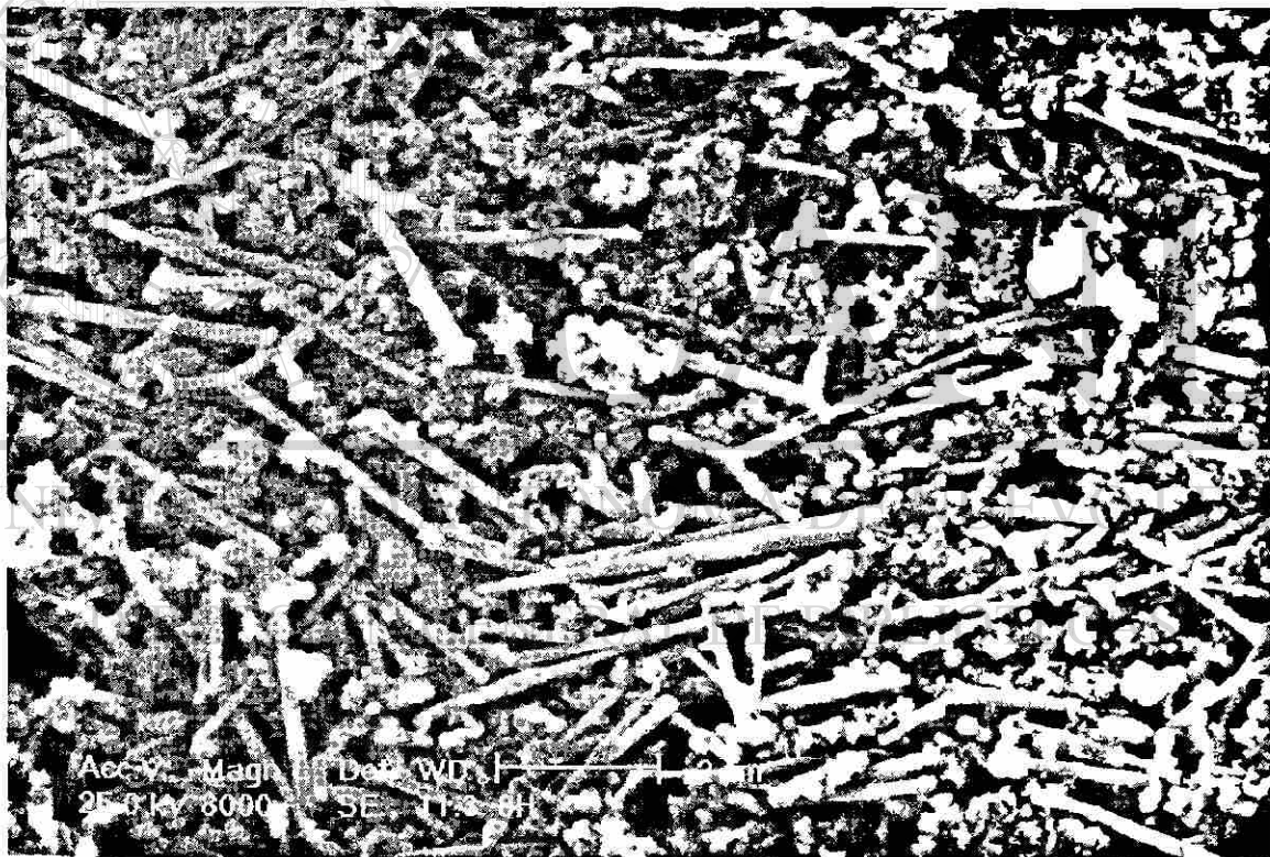
Fig. 5.16 Micrografía de electrones secundarios de whiskers de carburo de silicio.
