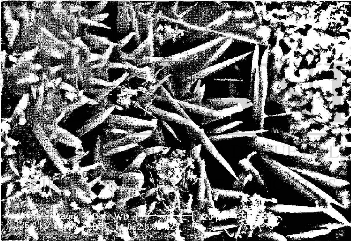
Fig. 5,43 Micrografía de whiskers embebidos en la fase líquida.
