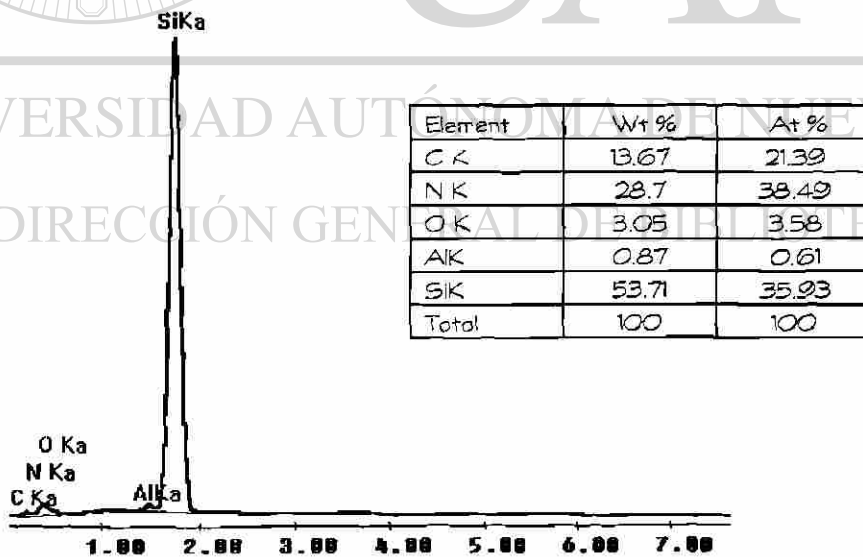
Fig. 5.34 EDS de la morfología en hélice.
