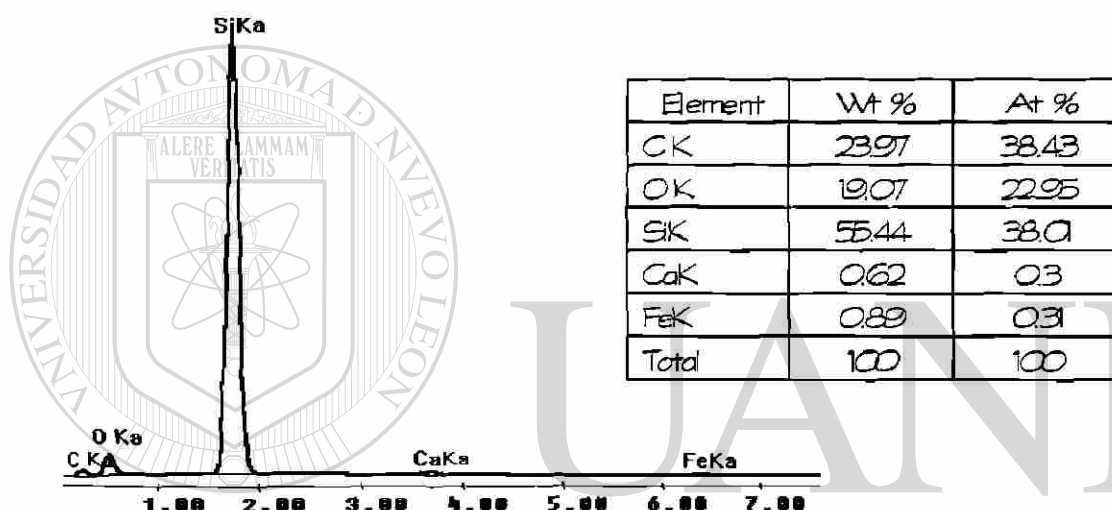
Fig. 5.15 Espectro de dispersión de energía de Rayos-X (EDS) de ceniza a 1400°C por 8 hrs.
