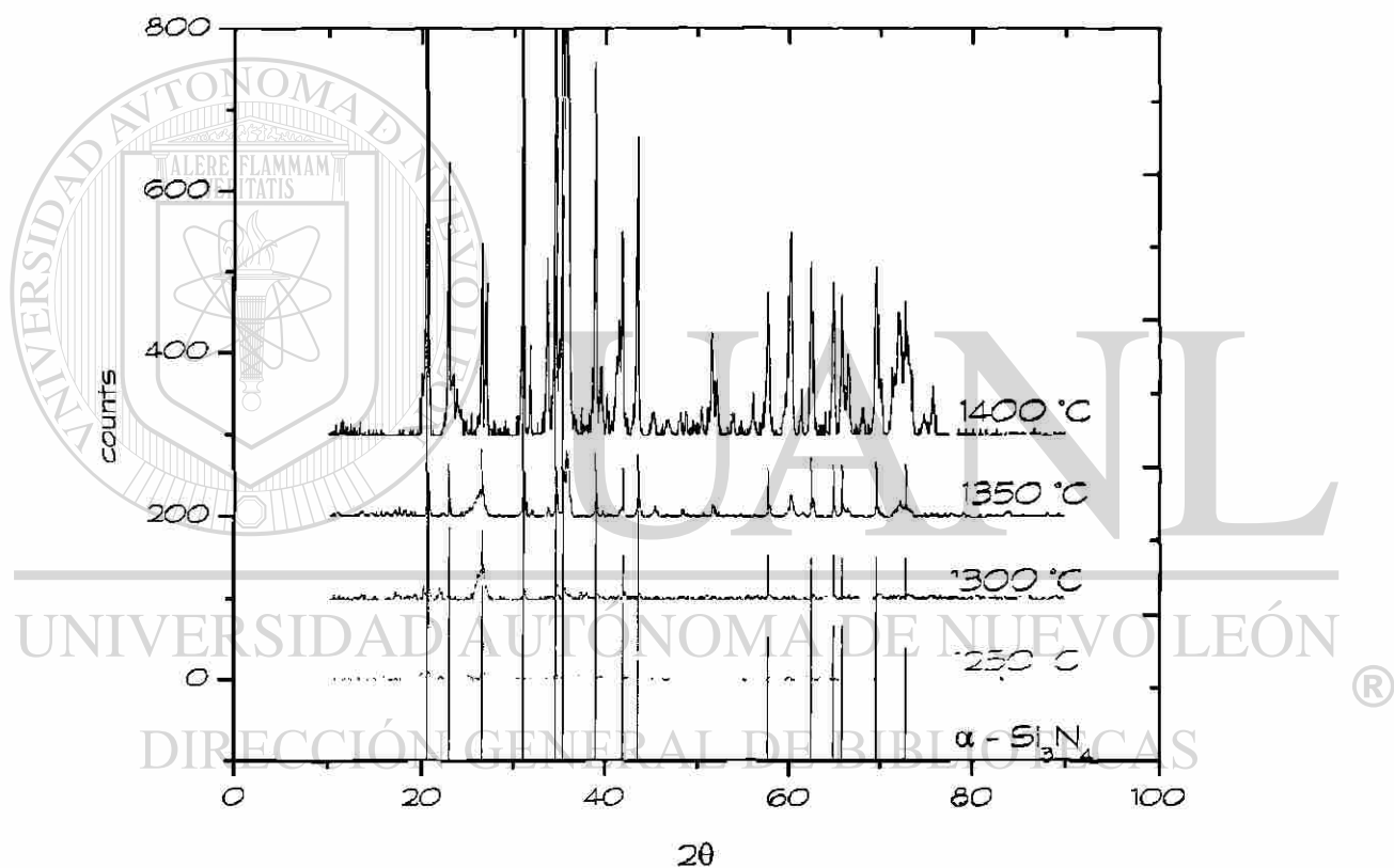
Fig. 5,10 Evolución de los difractogramas de las cenizas de cascarilla de arroz tratadas en atmósfera de nitrógeno por 6 horas.
