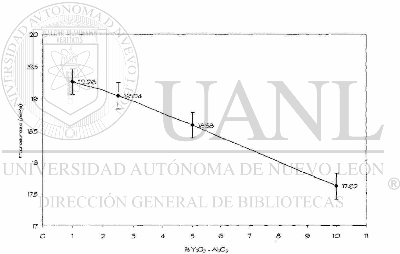
Fig. 5.54 Gráfico de microdureza vs. % de aditivos.
