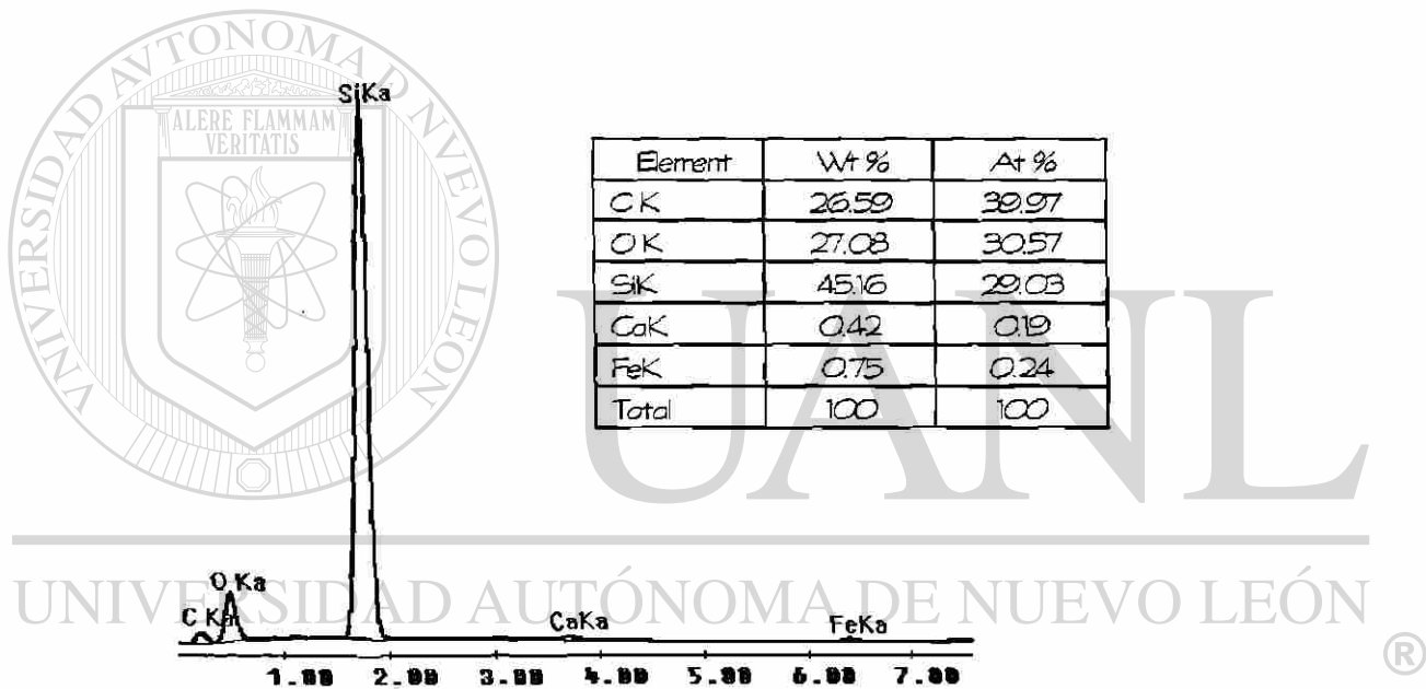
5,18 Espectro de Dispersión de Energía de Rayos X (EDS) de la parte interna de la cascarilla de arroz pirolizada a 1400°C por 8 horas.
