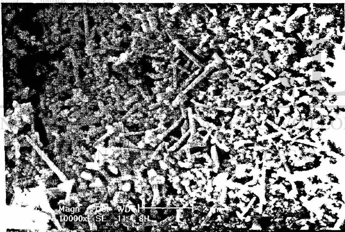
Fig. 5.17 Micrografía de electrones secundarios de la pared de la cascarilla de arroz pirolizada a 1400°C por 8 horas.
