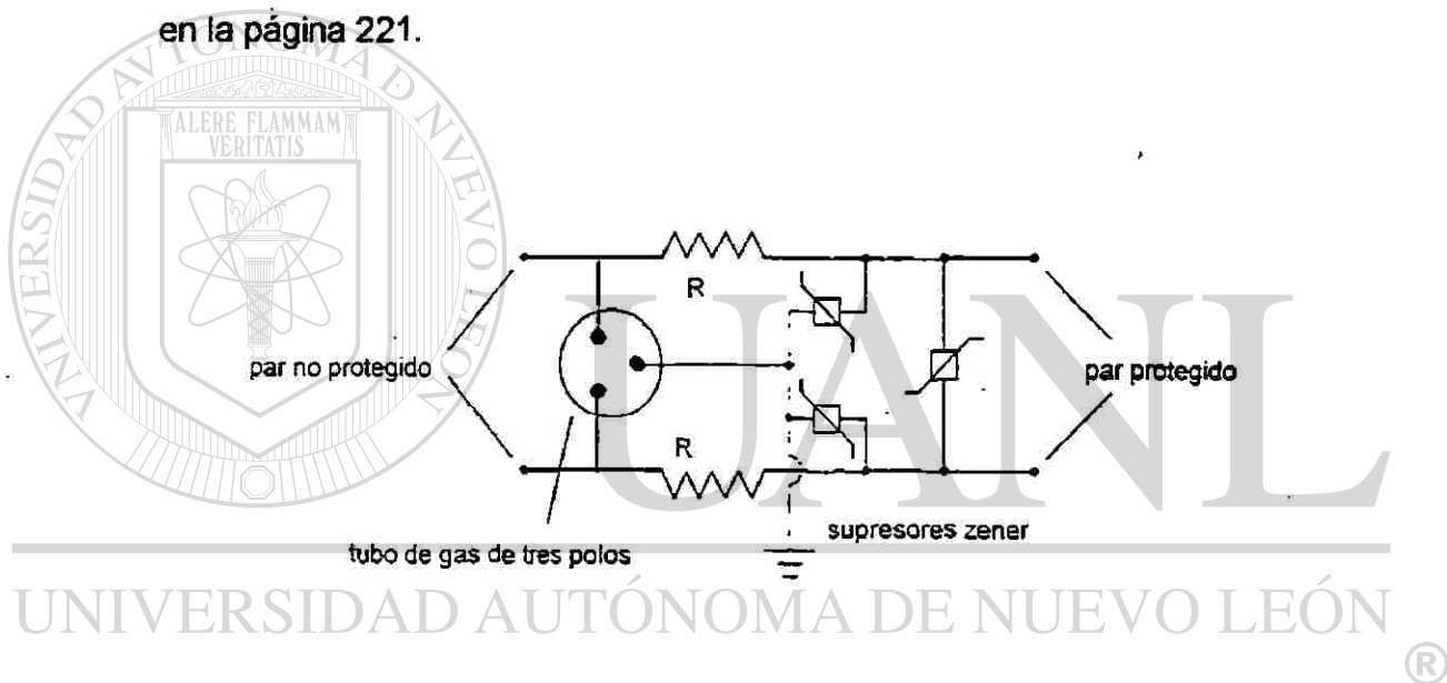
Figura 4 Supresor de sobrevoltajes transitorios para línea de datos.
