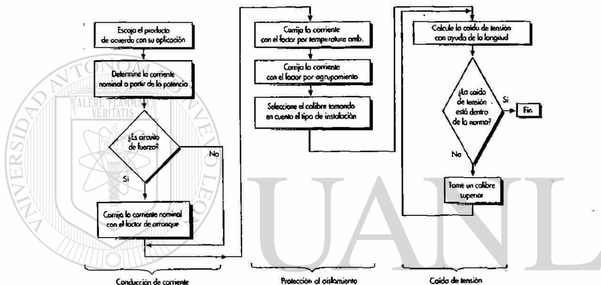
Pasos para calcular calibres mínimos
