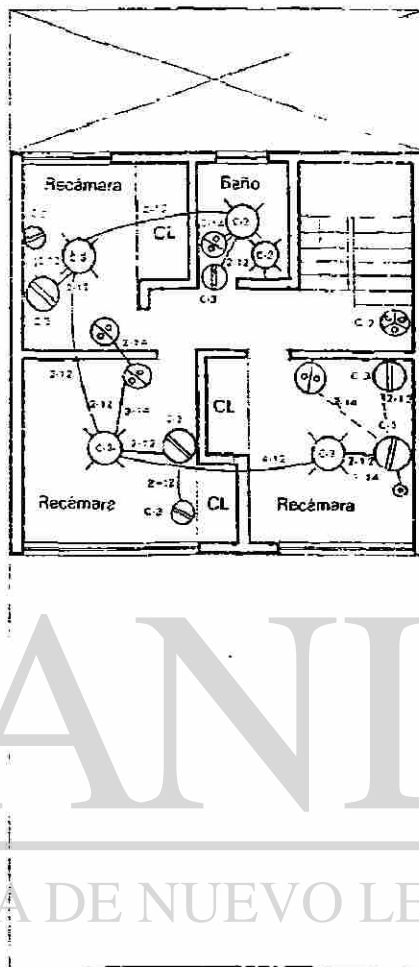
Planta alta
