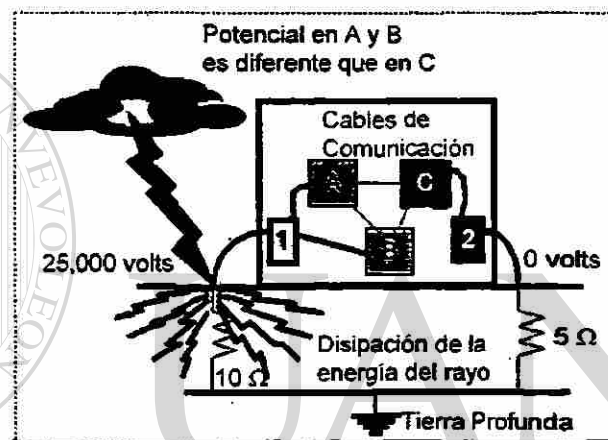
Figura 10. Electrodo aislados
