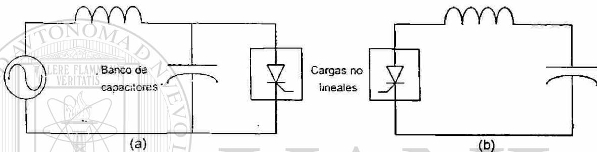
Figura. Circuitos que ejemplifican: (a) resonancia paralelo y (b) resonancia serie.
