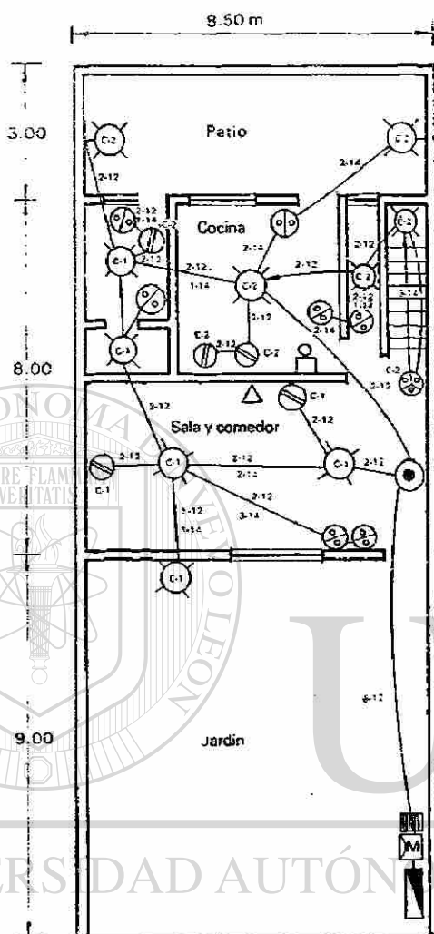
Planta baja
