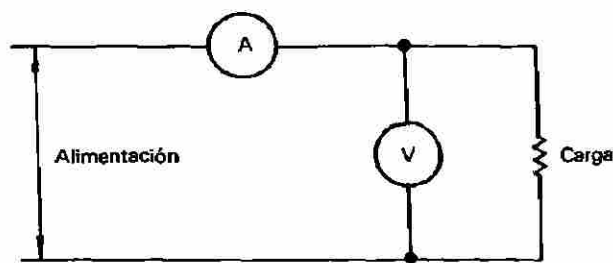
Cálculo de potencia con ampérmetro y voltímetro ( P = EI )
