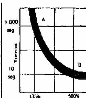
Porcentaje de la Corriente Nominal del interruptor
