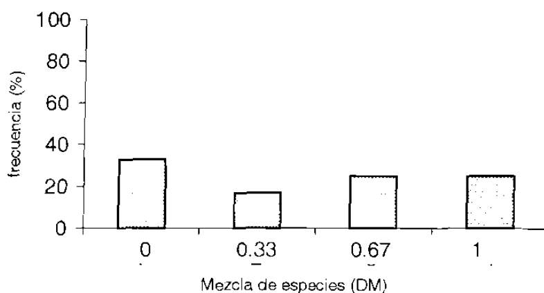
Figura 18: Índice de mezcla de especies.
