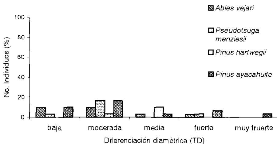
Figura 10: Índice de diferenciación diamétrica.
