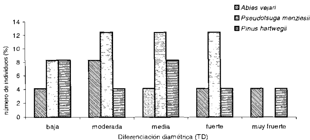
Figura 17: Índice de diferenciación diamétrica.
