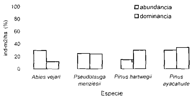
Figura 8: Abundancia y dominancia para la población del Cerro El Potosí.
