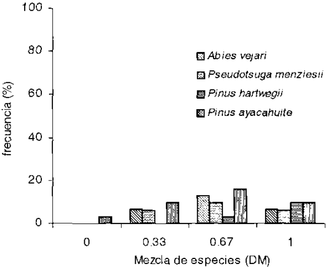
Figura 12: Grado de asociación del índice de mezcla de especies.
