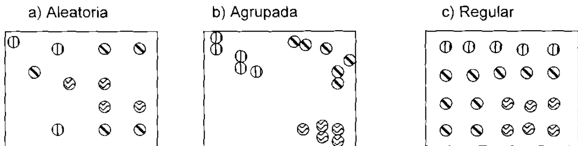
Figura 5: Tipos de distribución espacial.
