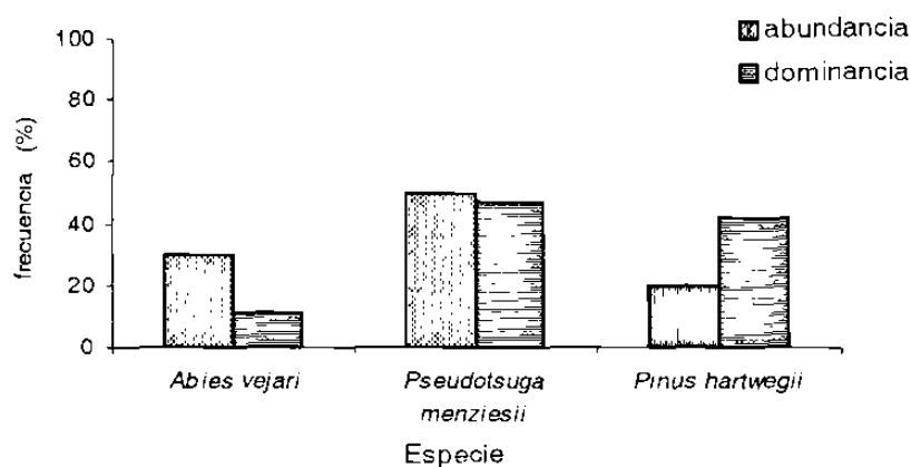
Figura 15: Abundancia y dominancia para la población en la Sierra La Marta.
