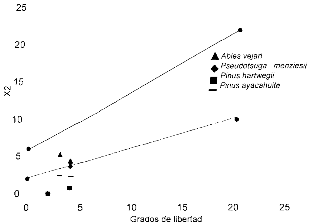
Figura 14: Distribución probabilística de las especies en función de X^2 .
