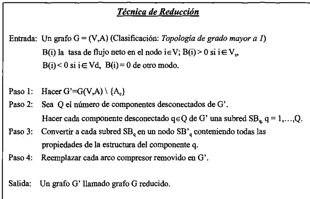
Figura 4.1: Algoritmo de la Técnica de Reducción aplicada a redes de gas natural.
