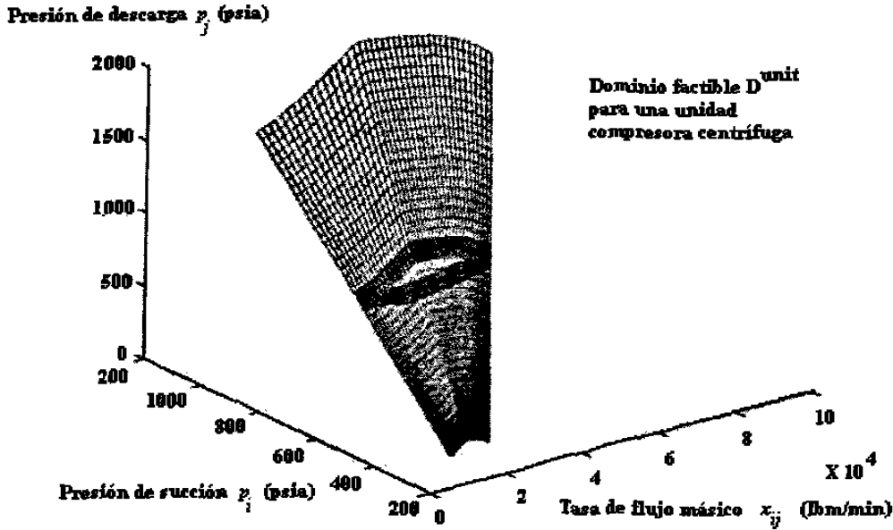
Figura 3.1: Dominio D^{unit}_{(ij)} de operación factible.
