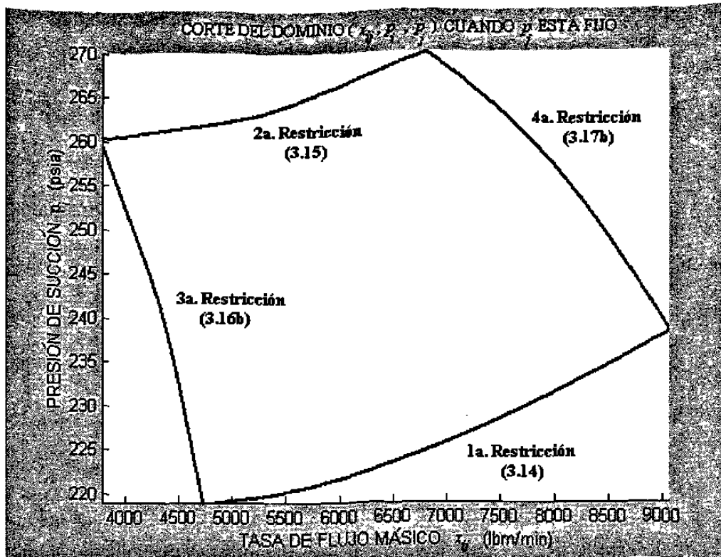
Figura 3.4: Frontera de operación factible D' definido por (3.14), (3.15), (3.16b) y (3.17b).
