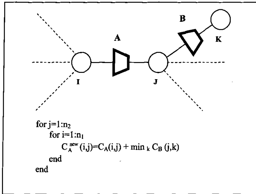
Figura 4.12: Combinación de dos compresores con un elemento colgante.
