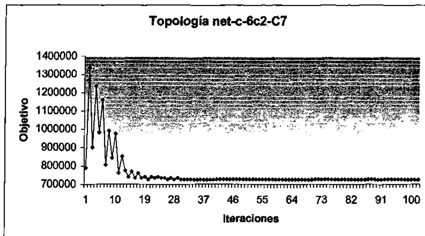
Figura 6.5: Convergencia de NONDP_TS en instancia net-c-6c2-C7.
