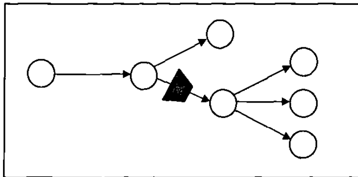
Figura 4.3: Reclasificación: Topología de grado 1.
