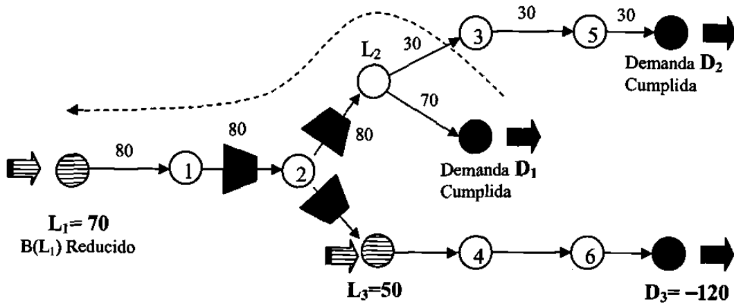
Figura 4.8: 2ª iteración del algoritmo de Asignación “clásica”.
