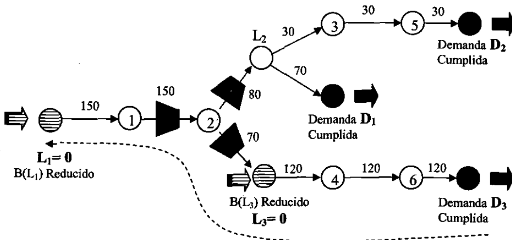
Figura 4.9: 3ª iteración del algoritmo de Asignación “clásica”.
