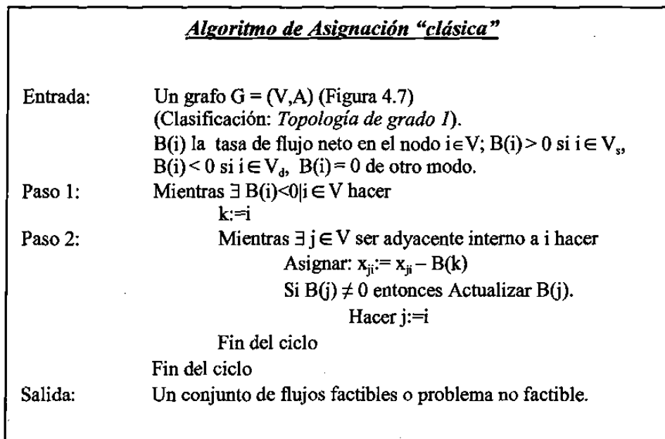
Figura 4.5: Algoritmo de Asignación “clásica”.
