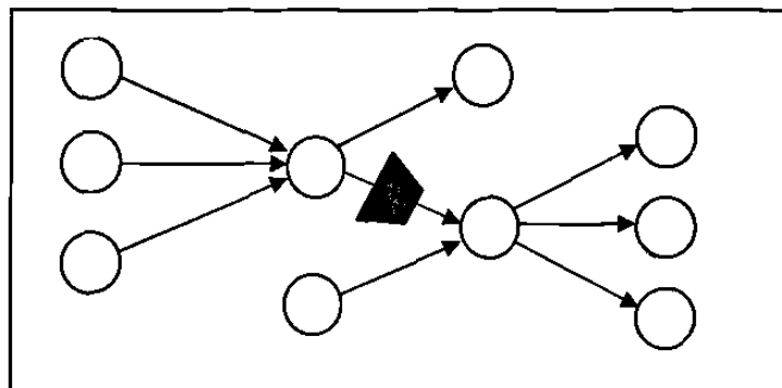
Figura 4.4: Reclasificación: Topología de grado mayor a 1.
