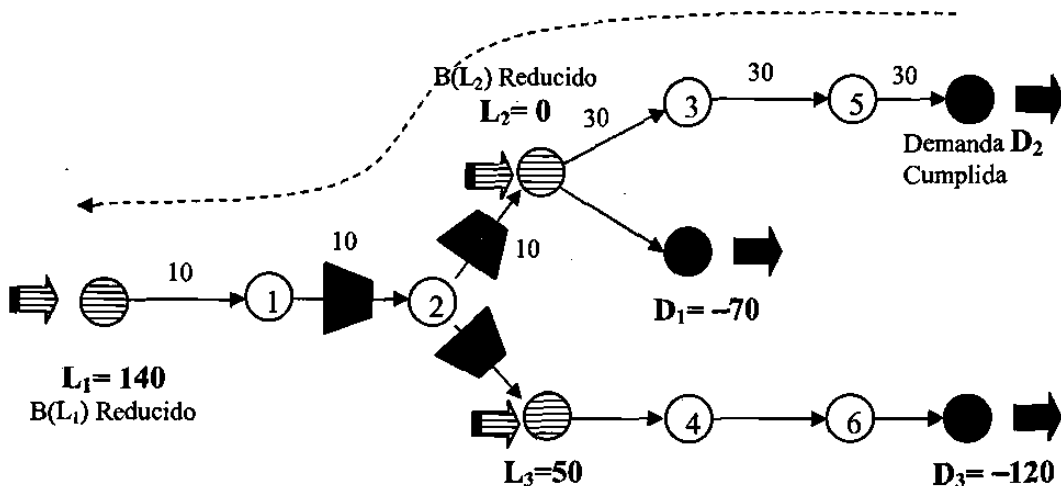
Figura 4.7: 1ª iteración del algoritmo de Asignación "clásica".
