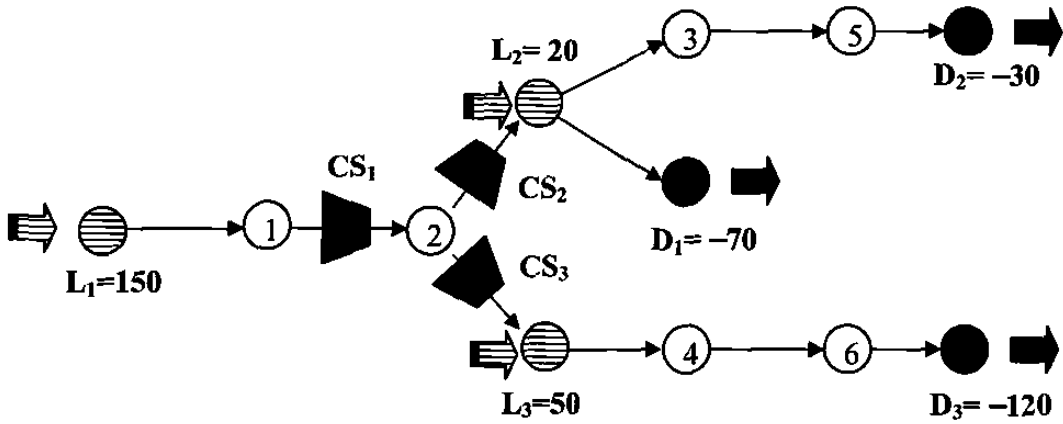
Figura 4.6: Grafo clasificado como topología de grado 1.
