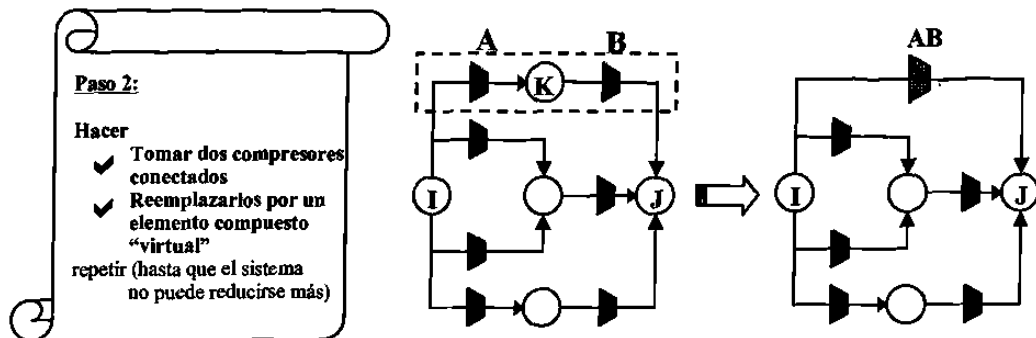
Figura 4.16: Ejecución del Paso 2 del algoritmo de DP no secuencial.
