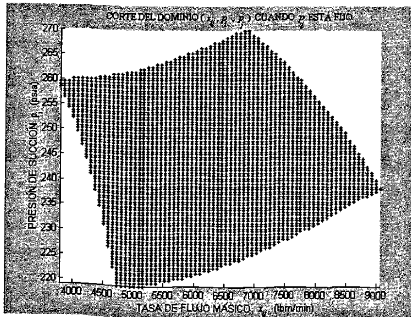
Figura 3.3: Superficie del dominio D_{(i,j)}^{unit} cuando p_j está fijo.
