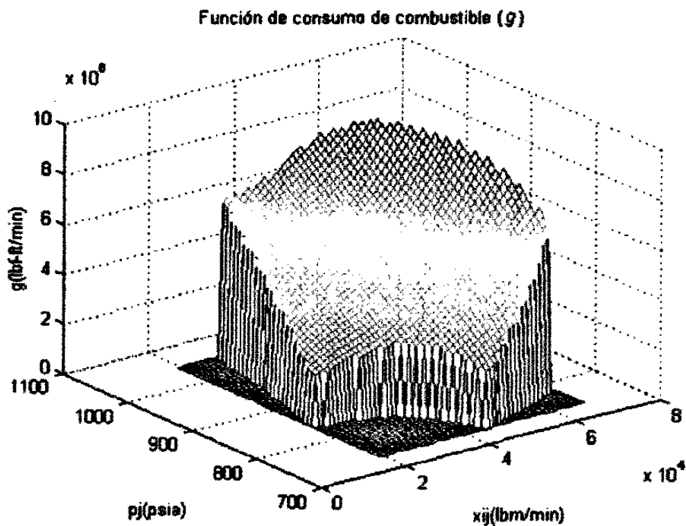
Figura 3.5: Gráfica de la función del consumo de combustible cuando p_i está fijo.
