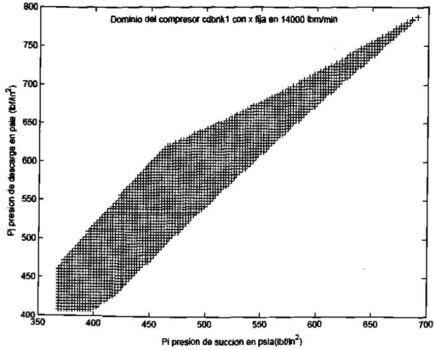
Figura 3.2: Gráfica del dominio D_{(i,j)}^{unit} cuando x_{ij} está fija.
