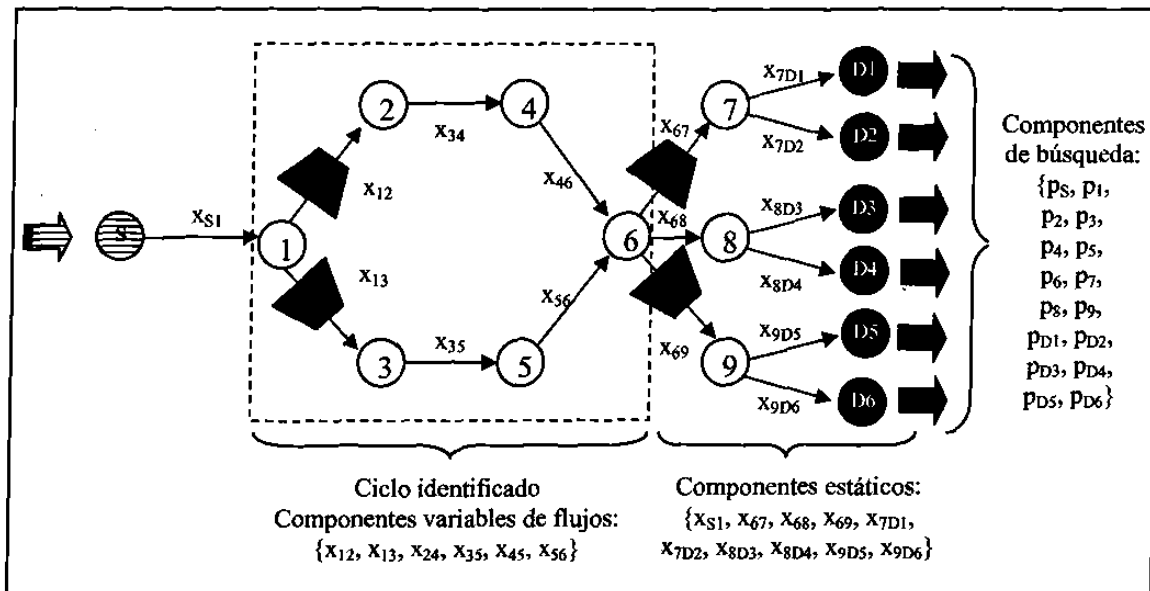
Figura 5.1: Topología cíclica en la cual se definen los tres componentes básicos de una solución factible en el procedimiento NONDP_TS.
