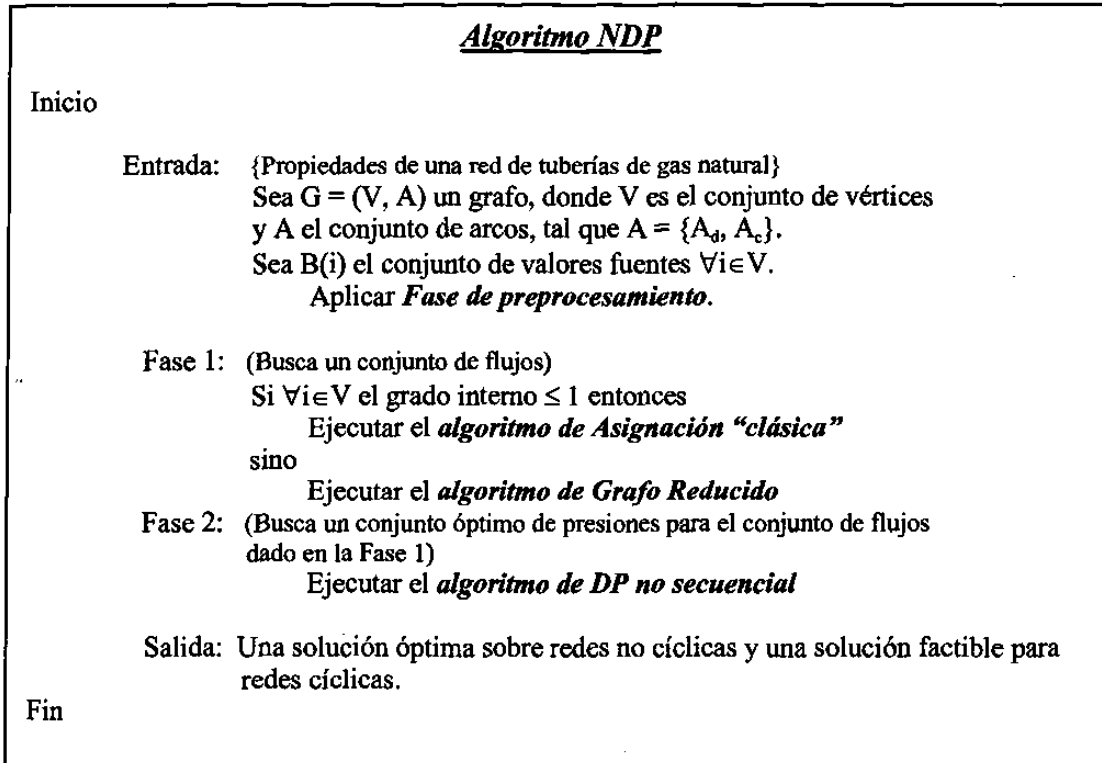
Figura 4.2: Algoritmo NDP para el PMCC.
