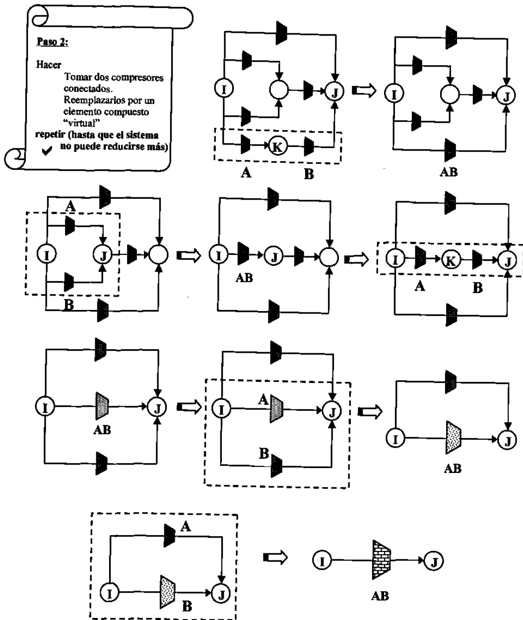
Figura 4.17: Reducción óptima de un sistema de red por la técnica de DP no secuencial.
