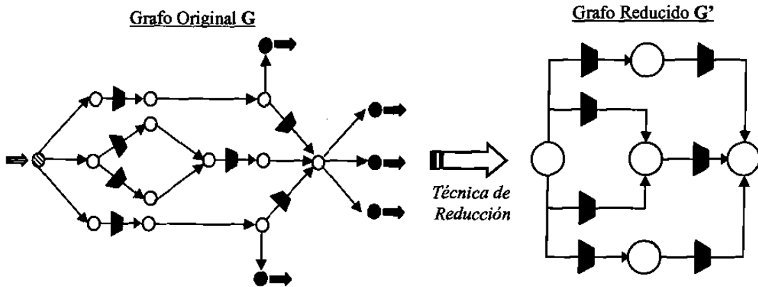
Figura 4.15: Grafo original G y su grafo reducido G' correspondiente.
