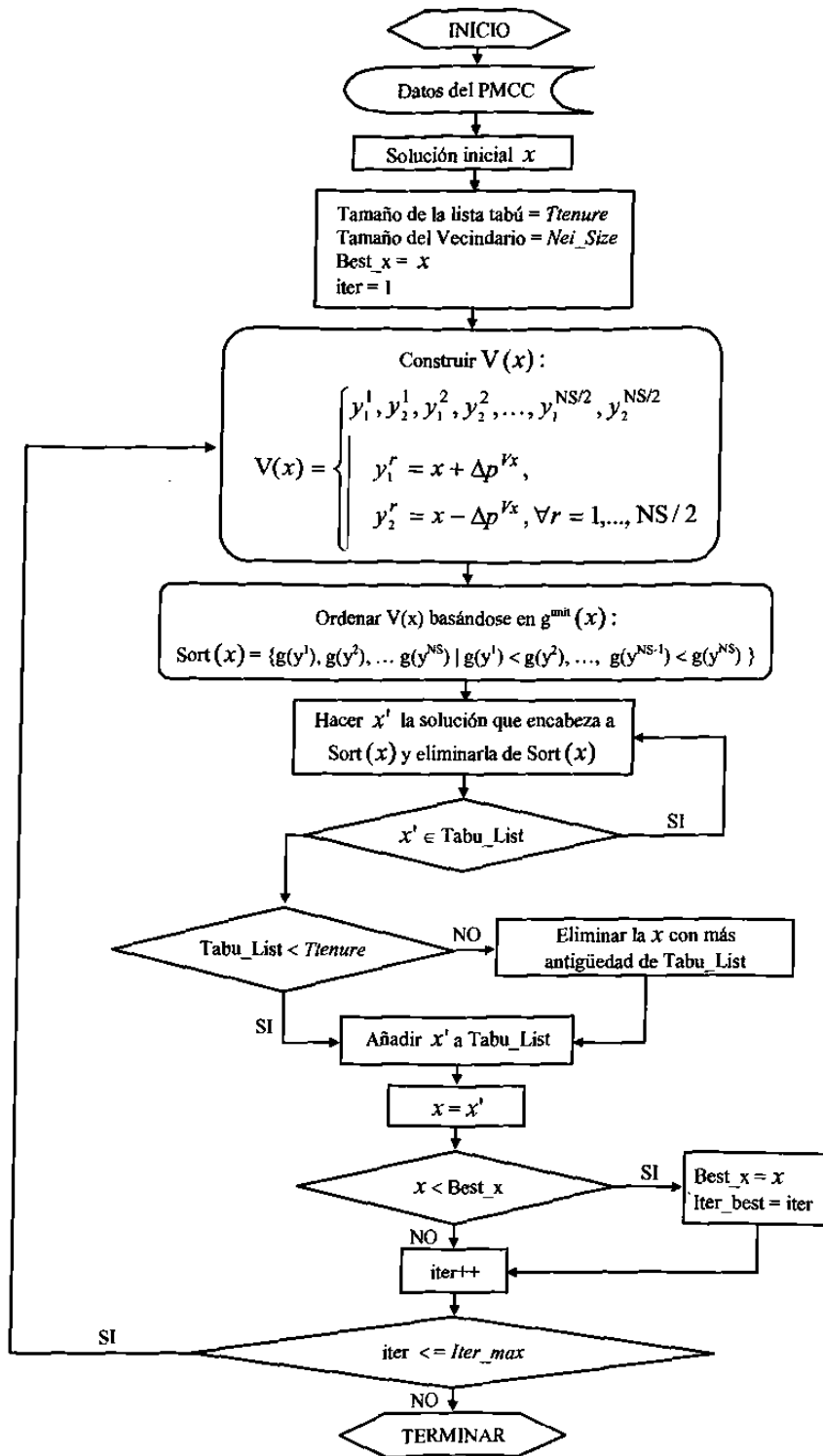
Figura 5.2: Diagrama de flujo del Algoritmo NONDP_TS.
