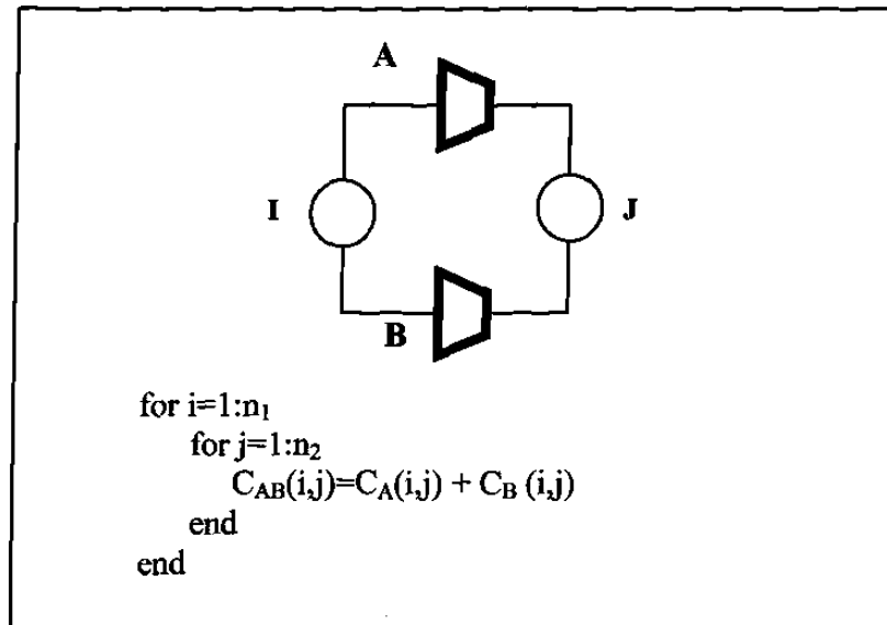
Figura 4.13: Combinación dos estaciones en paralelo.
