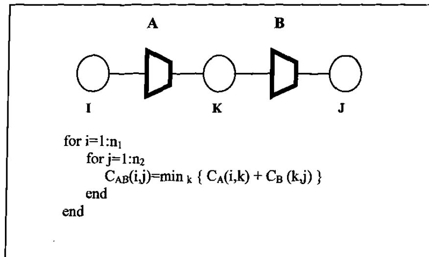
Figura 4.11: Combinación de dos estaciones en serie.
