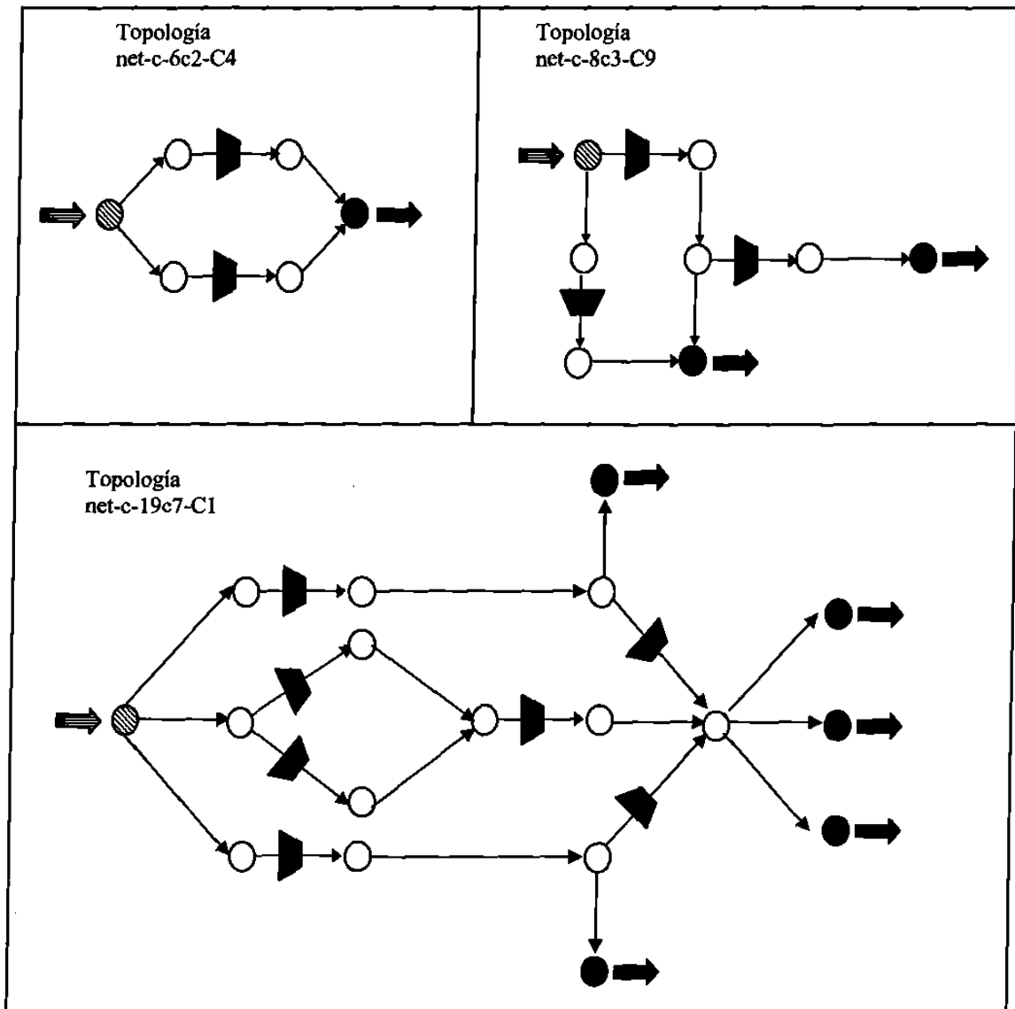
Figura 6.4: Ejemplos de instancias con estructuras cíclicas.
