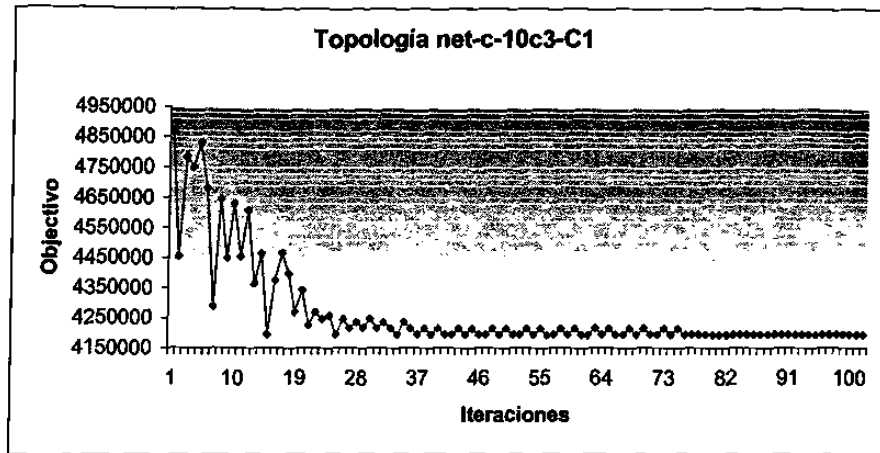
Figura 6.6: Convergencia de NONDP_TS en instancia net-c-10c3-C1.
