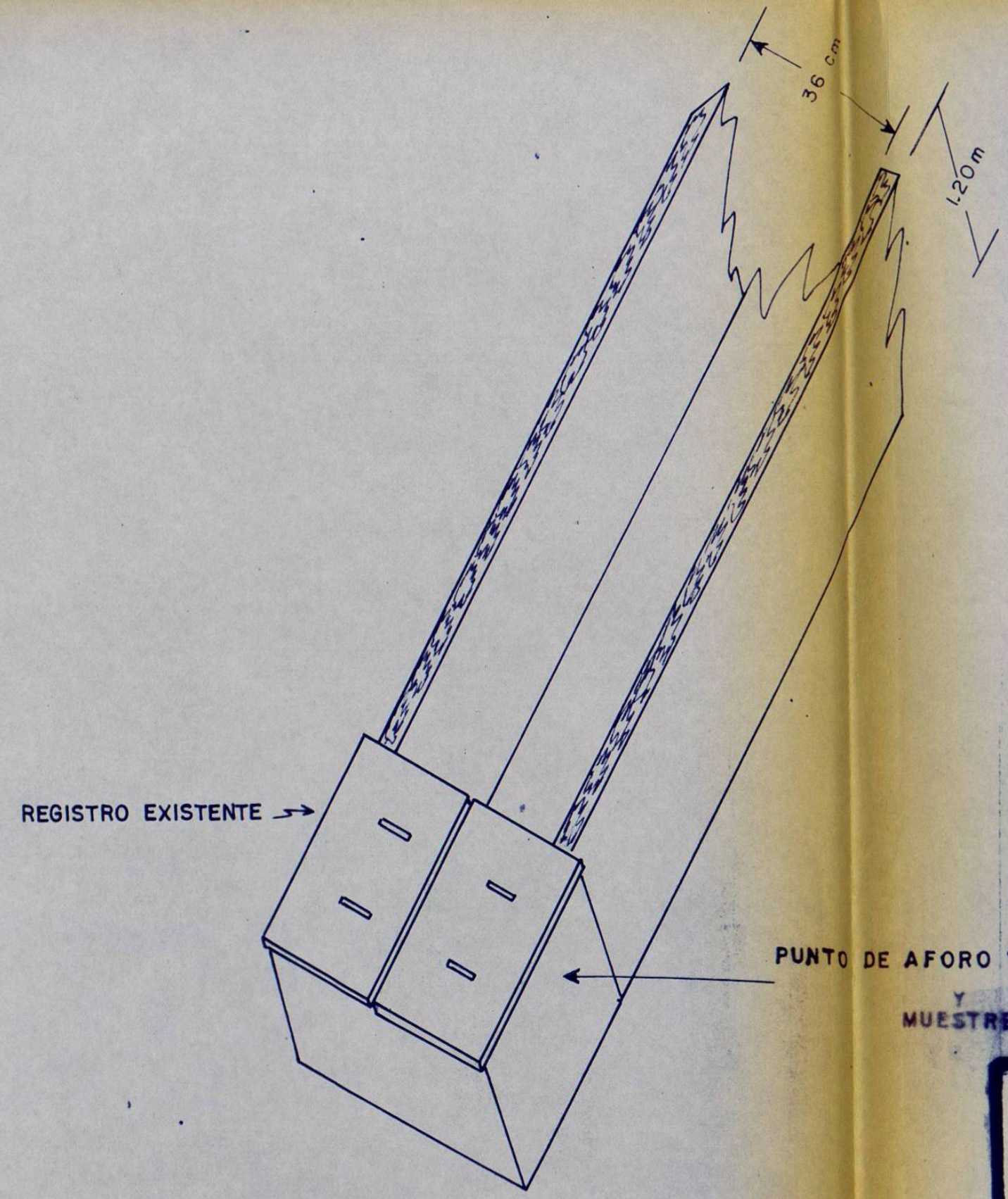
● DETALLE 3 SALIDA DEL DESARENADOR
