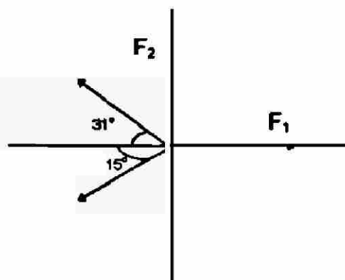
FIGURA 3.8 DIAGRAMA DE FUERZAS CASO 3
