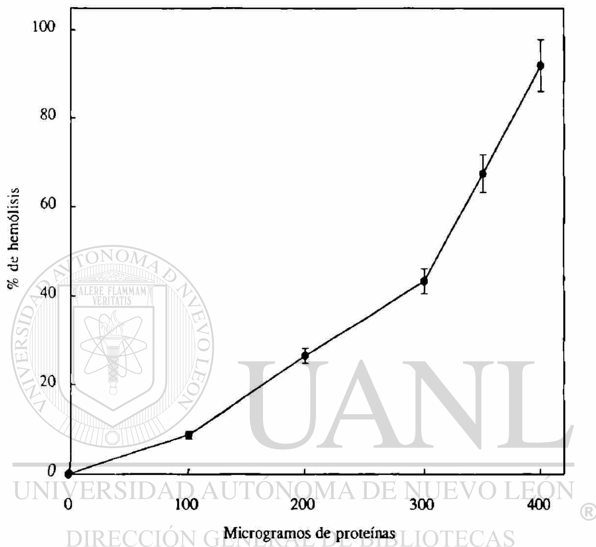
Figura 8. Curva dosis-respuesta de la fracción P30 de cepa HM1:IMSS crecida en PEHP-PACSR. Después de una hora de incubación a 37 °C, determinamos el porcentaje de hemólisis en mezclas de ensayo con 3 % de eritrocitos de rata y concentraciones variables de proteínas. Cada símbolo corresponde al promedio y desviación estándar de nueve determinaciones en tres experimentos independientes.
