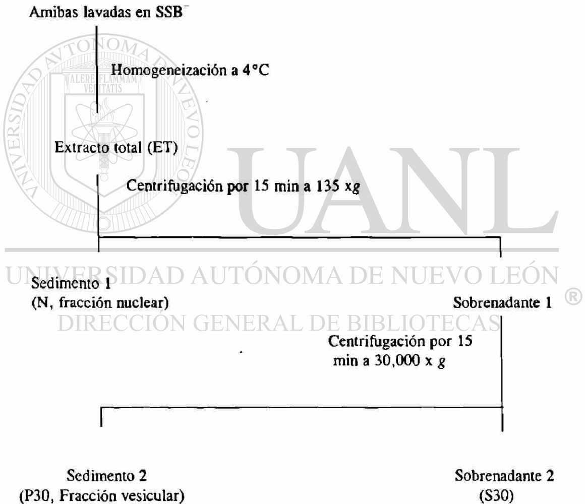
Figura 1. Obtención de las fracciones subcelulares amibianas (Saíd-Fernández y López-Revilla, 1982).
