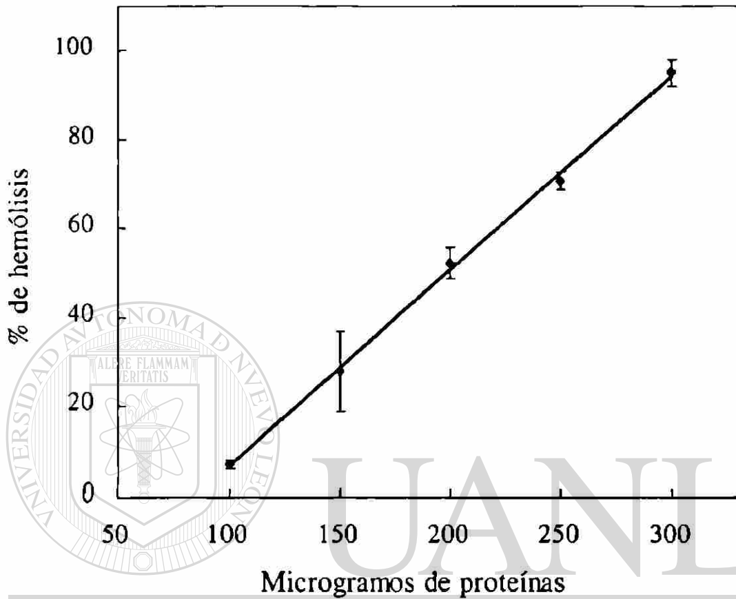
Figura 7. Curva dosis-respuesta de la fracción P30 de cepa HMI:IMSS crecida en PEHPS. Después de una hora de incubación a 37 °C, determinamos el porcentaje de hemólisis en mezclas de ensayo con 3 % de eritrocitos de rata y concentraciones variables de proteínas. Cada símbolo corresponde al promedio y desviación estándar de nueve determinaciones en tres experimentos independientes.
