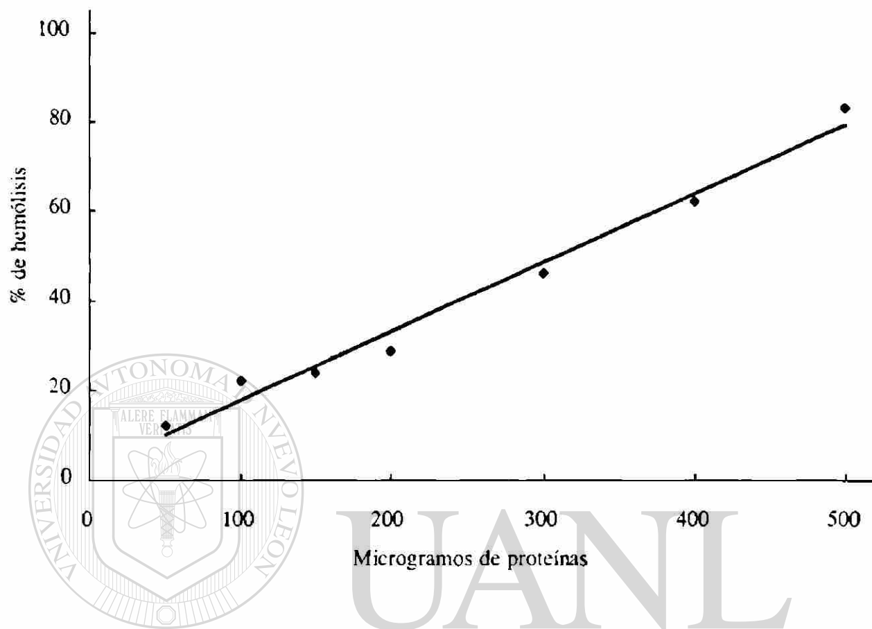
Figura 9. Curva dosis-respuesta de la fracción P30 de cepa HMI:IMSS crecida en PEHP-LIPO. Después de una hora de incubación a 37 °C, determinamos el porcentaje de hemólisis en mezclas de ensayo con 3 % de eritrocitos de rata y concentraciones variables de proteínas. Cada símbolo corresponde al promedio y desviación estándar de nueve determinaciones en tres experimentos independientes.
