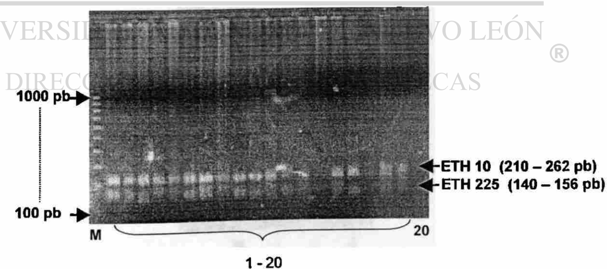
Figura 9. Verificación de Amplificación del múltiple 2 en Gel de Agarosa al 2%
