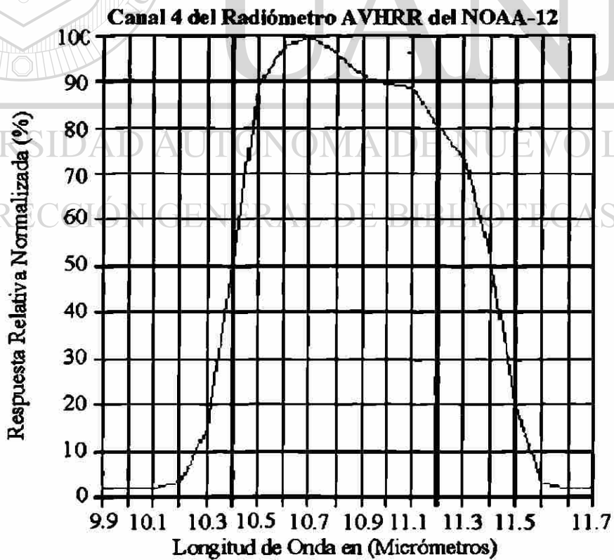
Figura 3.8 Curva de respuesta espectral de la banda 4 del sensor AVHRR del NOAA-12
