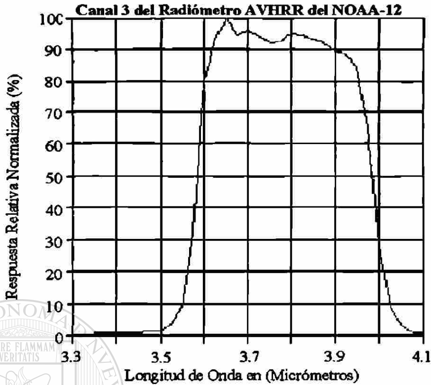
Figura 3.7 Curva de respuesta espectral de la banda 3 del sensor AVHRR del NOAA-12
