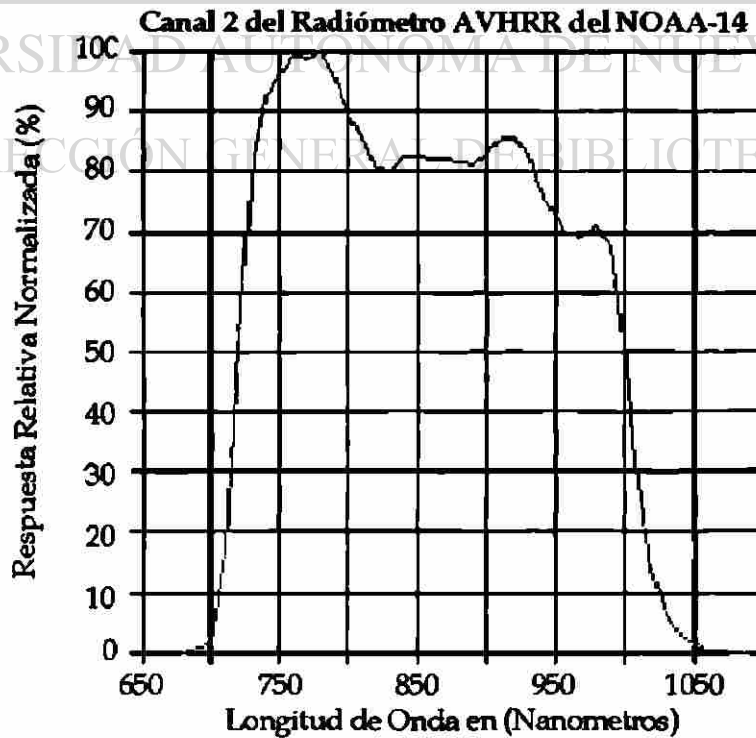
Figura 3.11 Curva de respuesta espectral de la banda 2 del sensor AVHRR del NOAA-14
