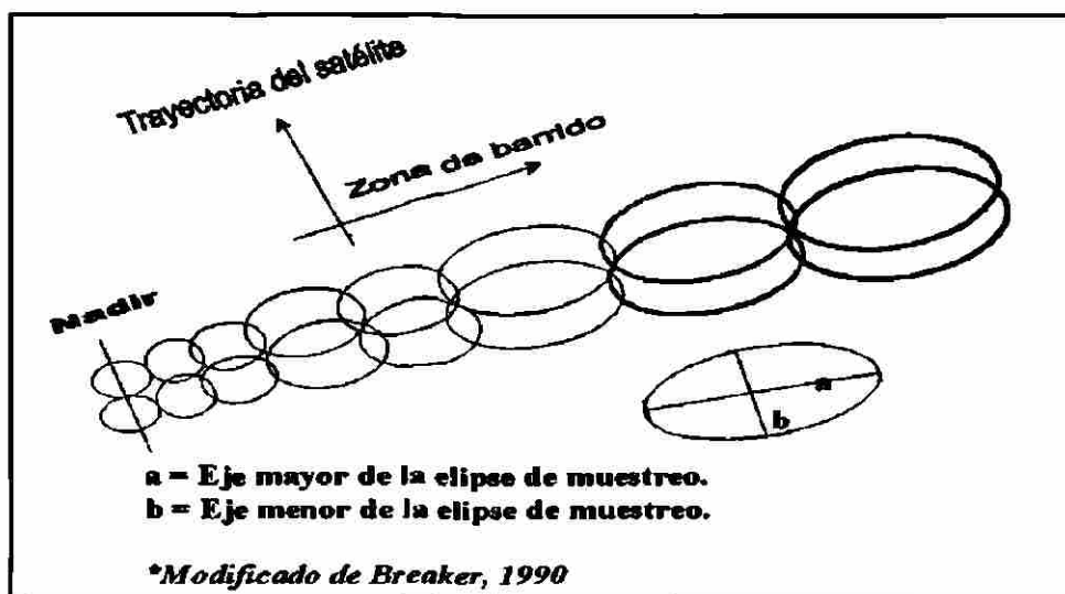
Figura 3.3 Geometría de un píxel de AVHRR y su deformación del nadir.
