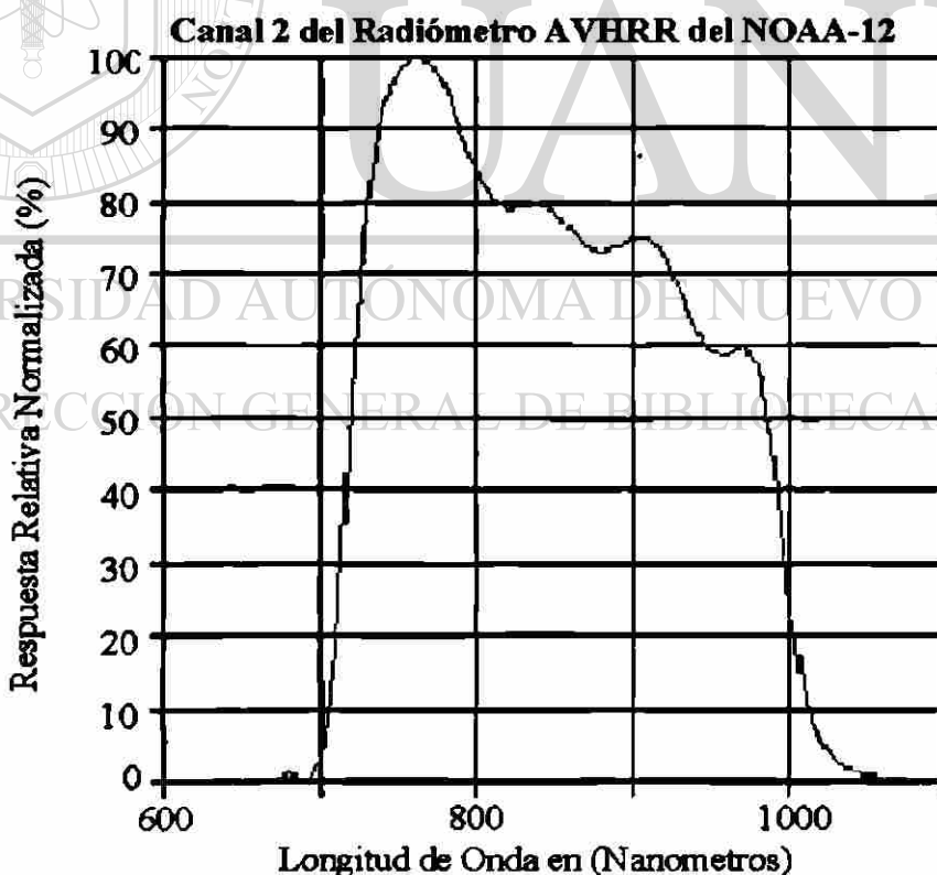
Figura 3.6 Curva de respuesta espectral de la banda 2 del sensor AVHRR del NOAA-12
