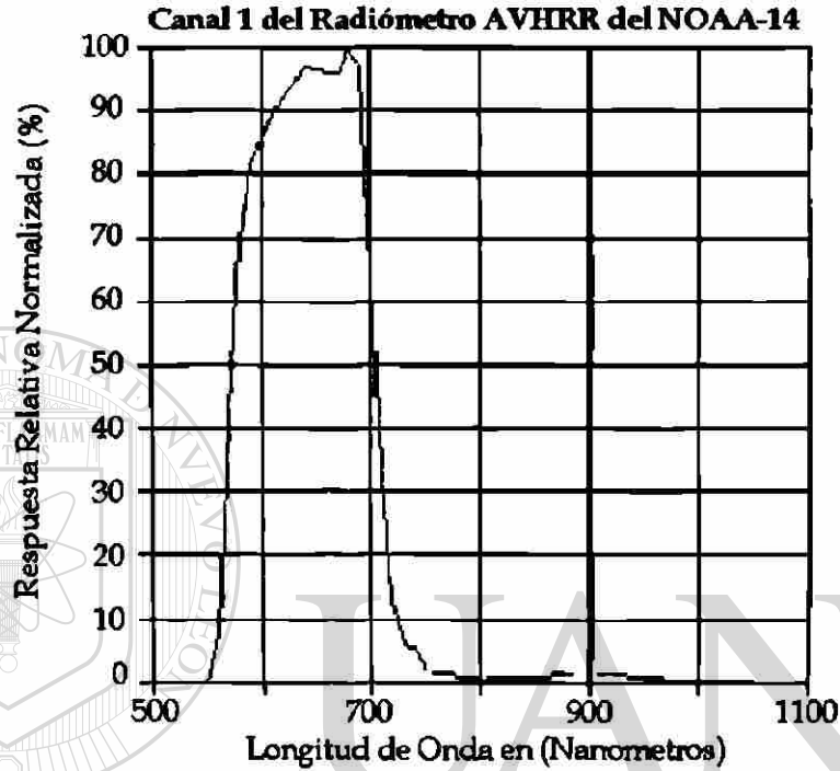
Figura 3.10 Curva de respuesta espectral de la banda 1 del sensor AVHRR del NOAA-14
