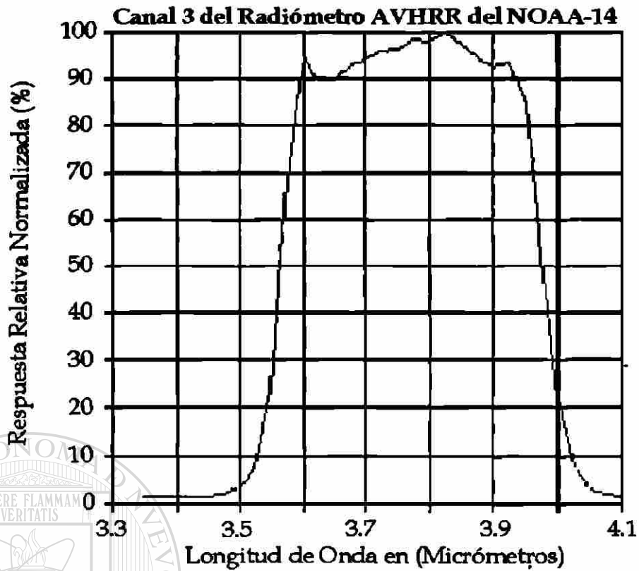
Figura 3.12 Curva de respuesta espectral de la banda 3 del sensor AVHRR del NOAA-14
