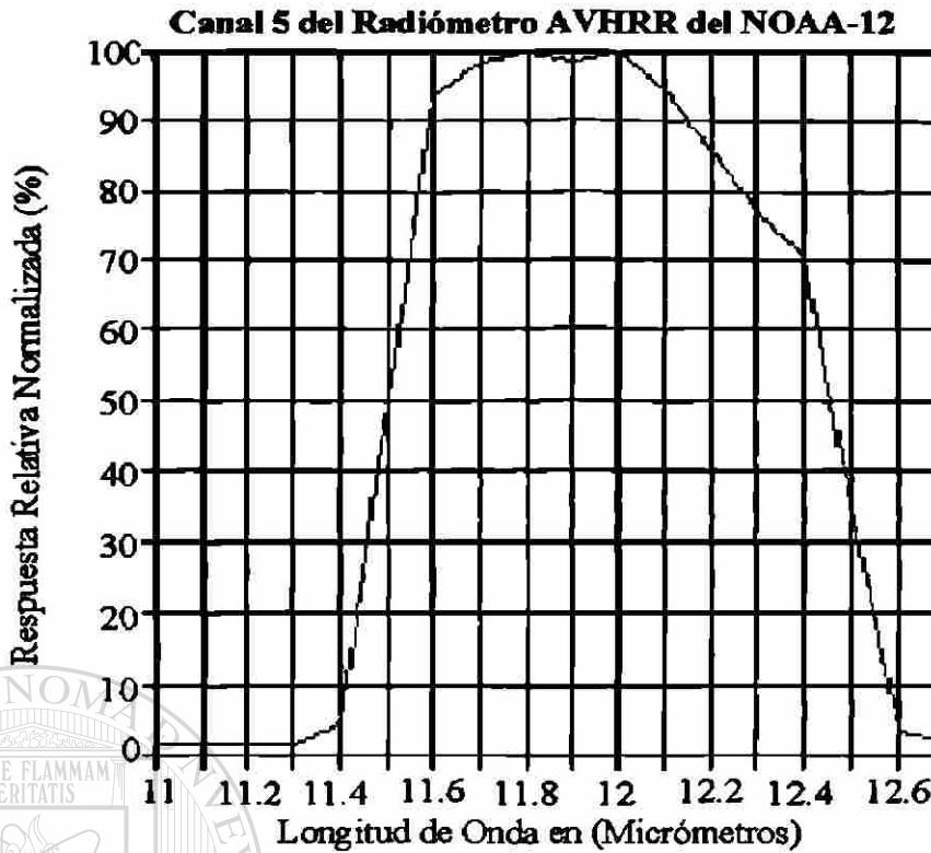
Figura 3.9 Curva de respuesta espectral de la banda 5 del sensor AVHRR del NOAA-12
