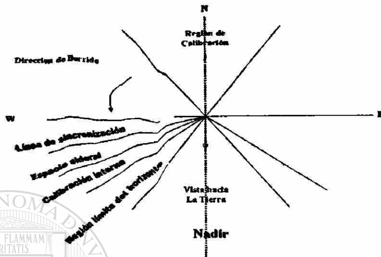
Figura 3.2 Dirección de barrido del espejo del radiómetro AVHRR
