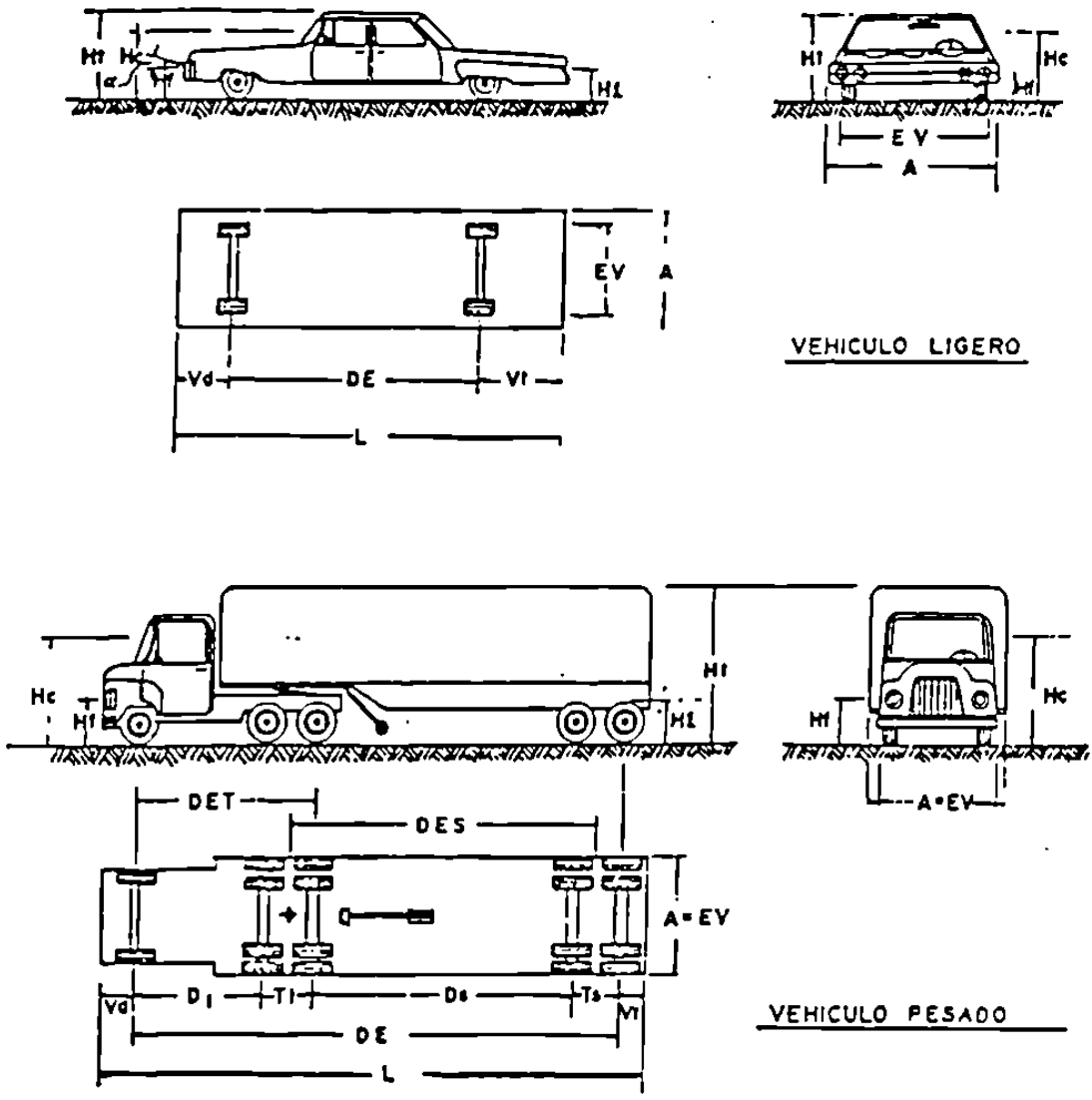
Figura 2. Dimensiones de los vehículos ligeros y pesados
