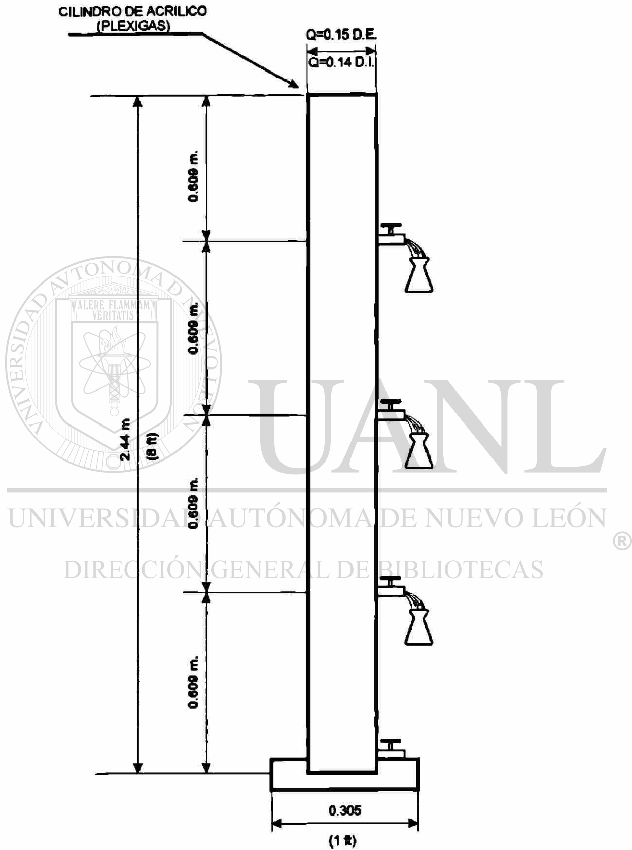
FIG. N° 4.2 MODELO DE LABORATORIO DE COLUMNA DE SEDIMENTACIÓN DE PARTÍCULAS FLOCULENTAS
