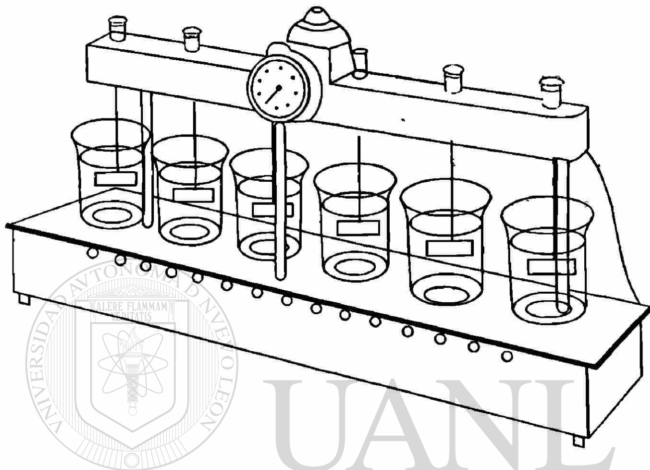
FIG. N° 4.7 EXPERIMENTAL DE PRUEBA DE JARRAS PARA OBTENER DOSIS ÓPTIMA DE COAGULANTES
