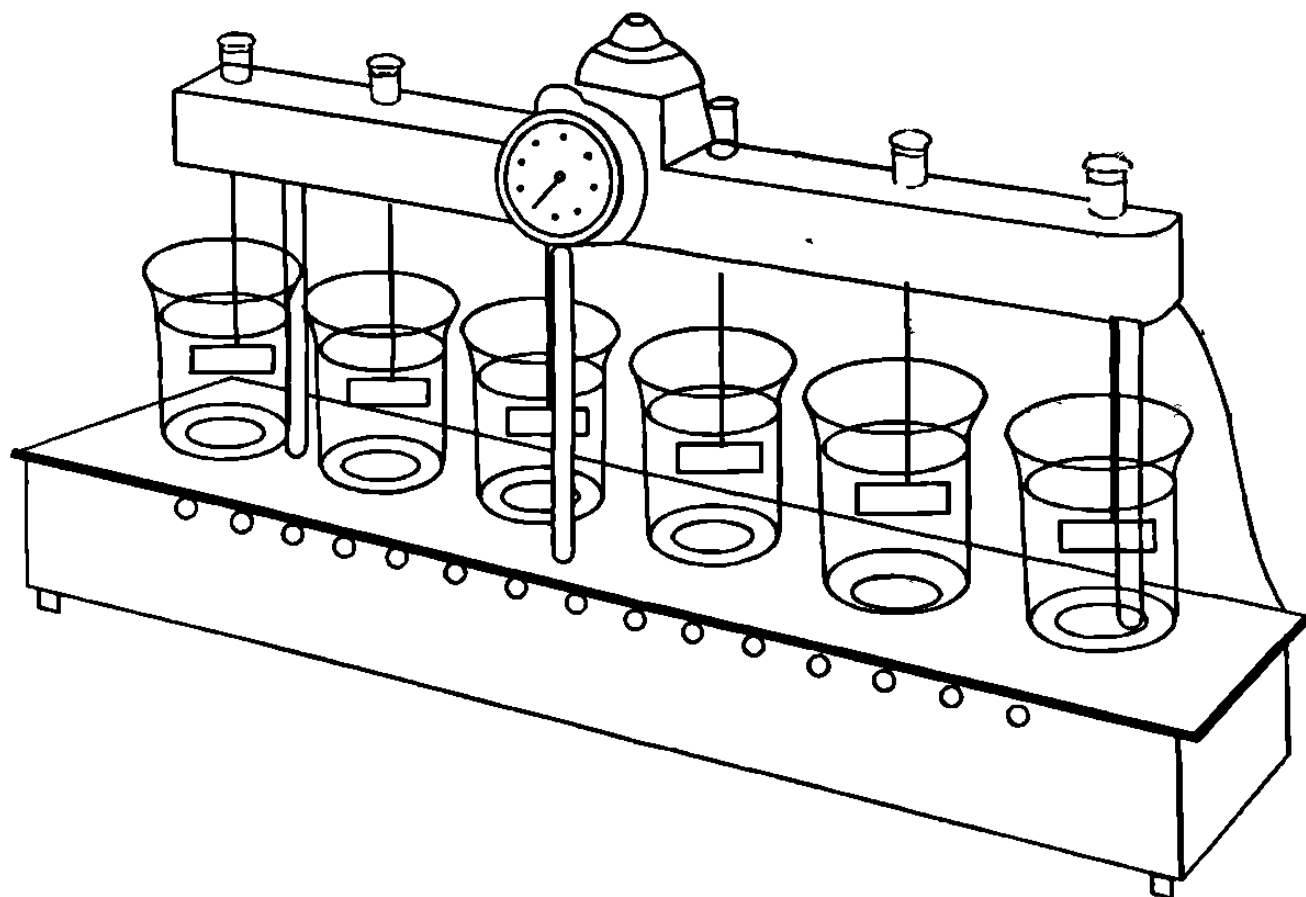
FIG. N° 4.7 EXPERIMENTAL DE PRUEBA DE JARRAS PARA OBTENER DOSIS ÓPTIMA DE COAGULANTES
