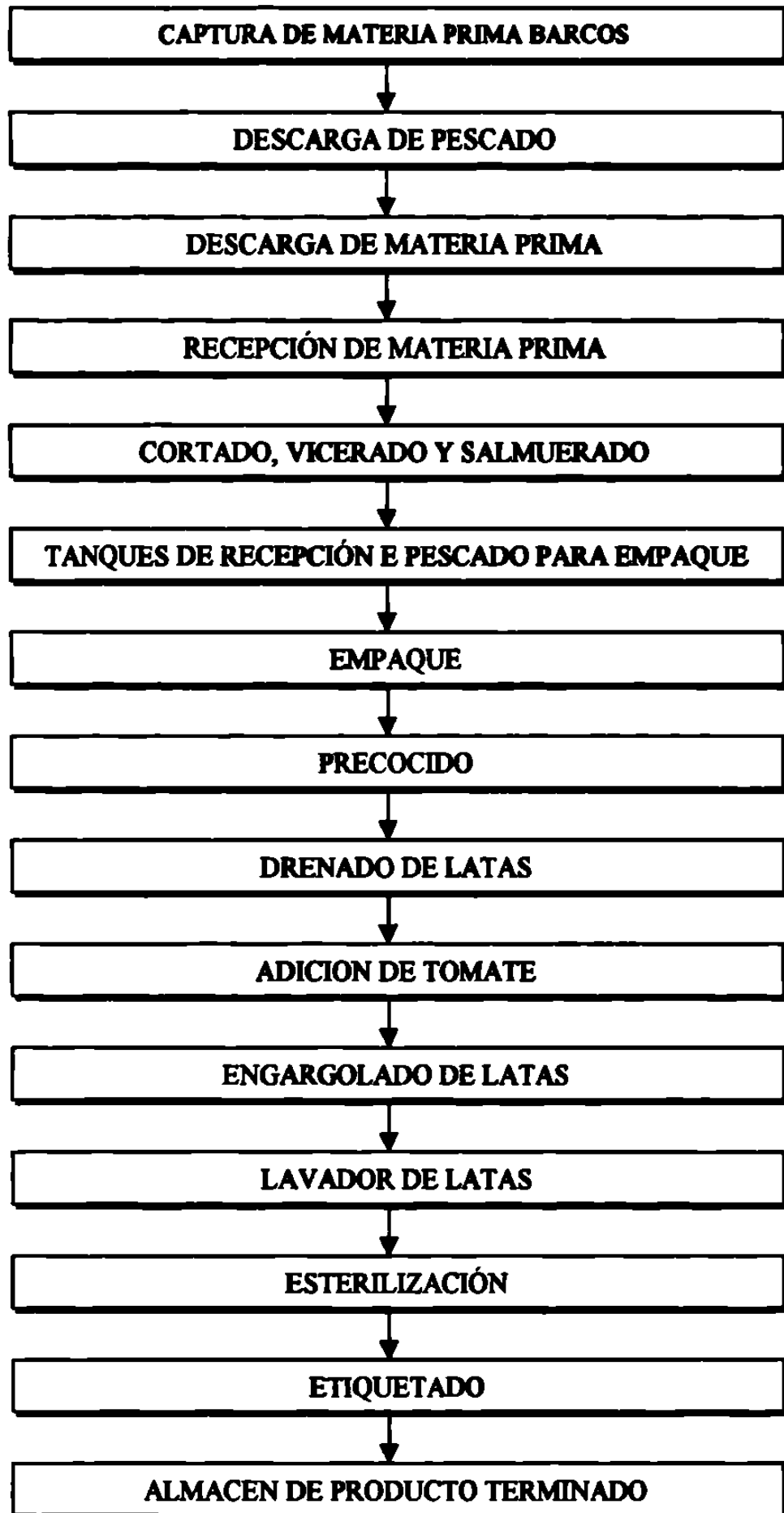
FIG. N° 2 DIAGRAMA GENERAL PARA ENLATADO DE SARDINA
