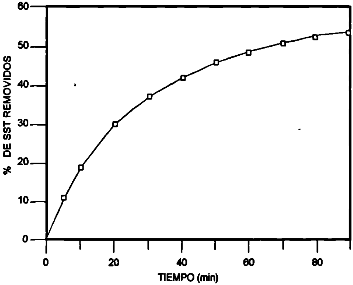
FIG. 4.11 Sedimentación floculenta industria enlatadora de pescado
