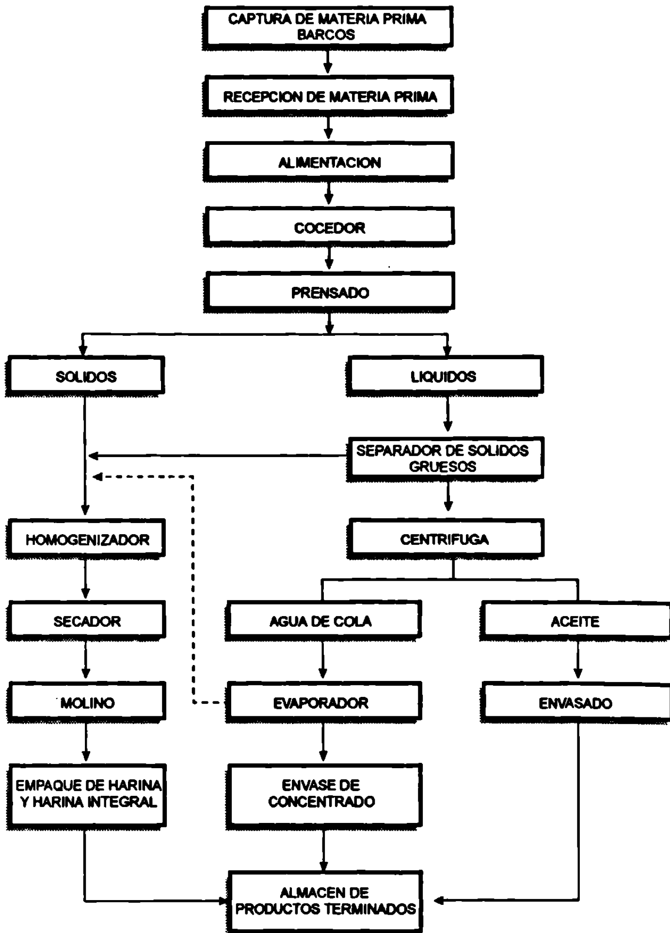
FIG. Nº 23 DIAGRAMA GENERAL PARA LA OBTENCIÓN DE HARINA DE PESCADO
