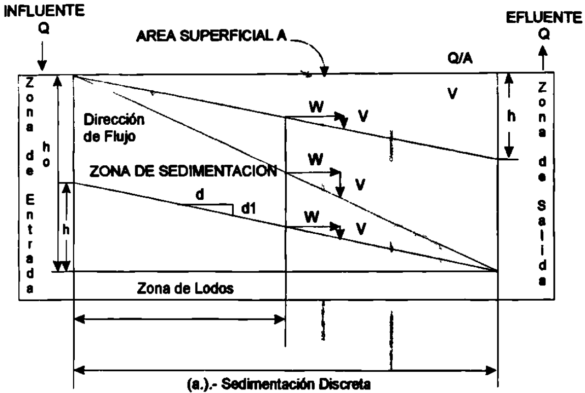
FIG. N° 4.1 TRAYECTORIA DE SEDIMENTACIÓN EN UN TANQUE DE SEDIMENTACION IDEAL
