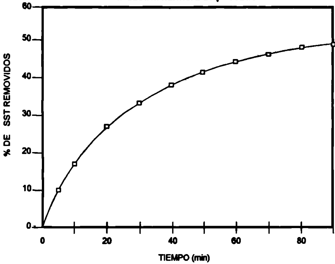
FIG.4.8. Sedimentación flocculenta Industria harinera de pescado
