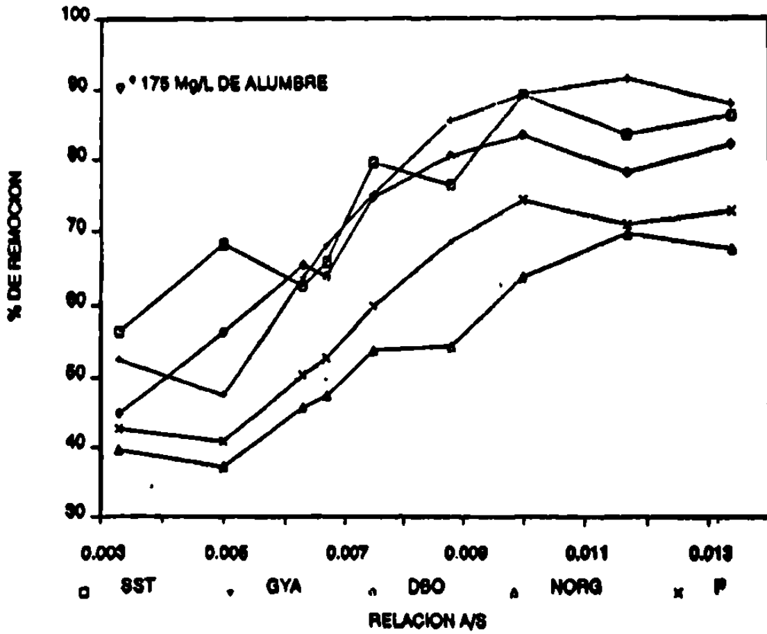
FIG. N° 4.14 FLOTACIÓN CON COAGULANTES INDUSTRIA ENLATADORA DE PESCADO
