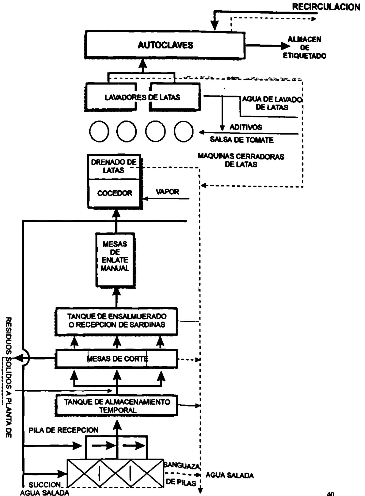
FIG. Nº 2.2 PROCESO DE ENLATADO DE ANCHOVETA
