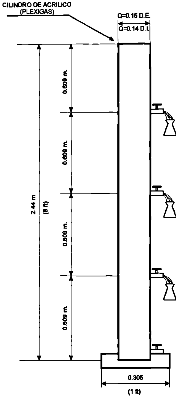
FIG. N° 4.2 MODELO DE LABORATORIO DE COLUMNA DE SEDIMENTACIÓN DE PARTÍCULAS FLOCULENTAS
