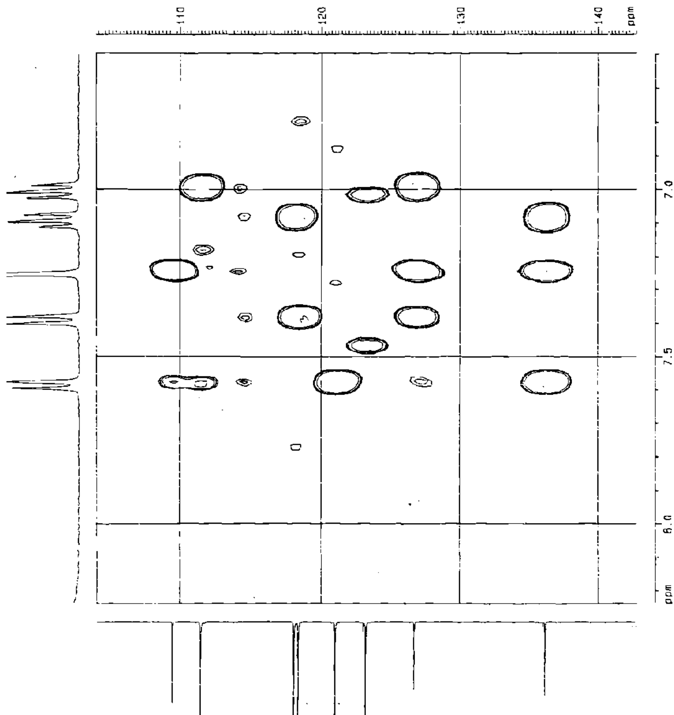
Fig. 33. Espectro de HMBC, del hidrocloreuro de triptamina
