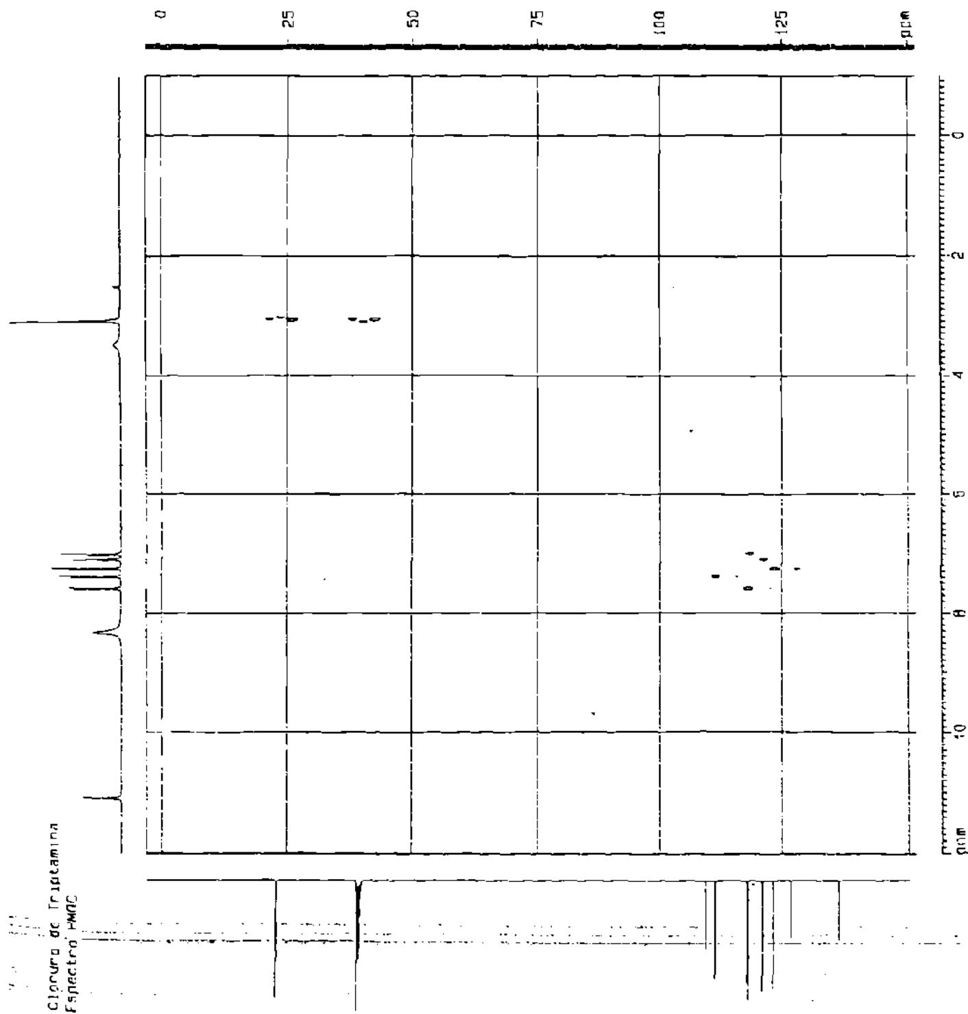
Fig. 28. Espectro de HMOC, del hidrocloreuro de triptamina
