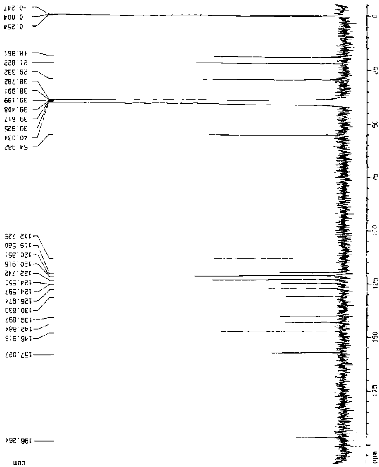
Fig. 44. Espectro de ^{13}\text{C} RMN, de 24
