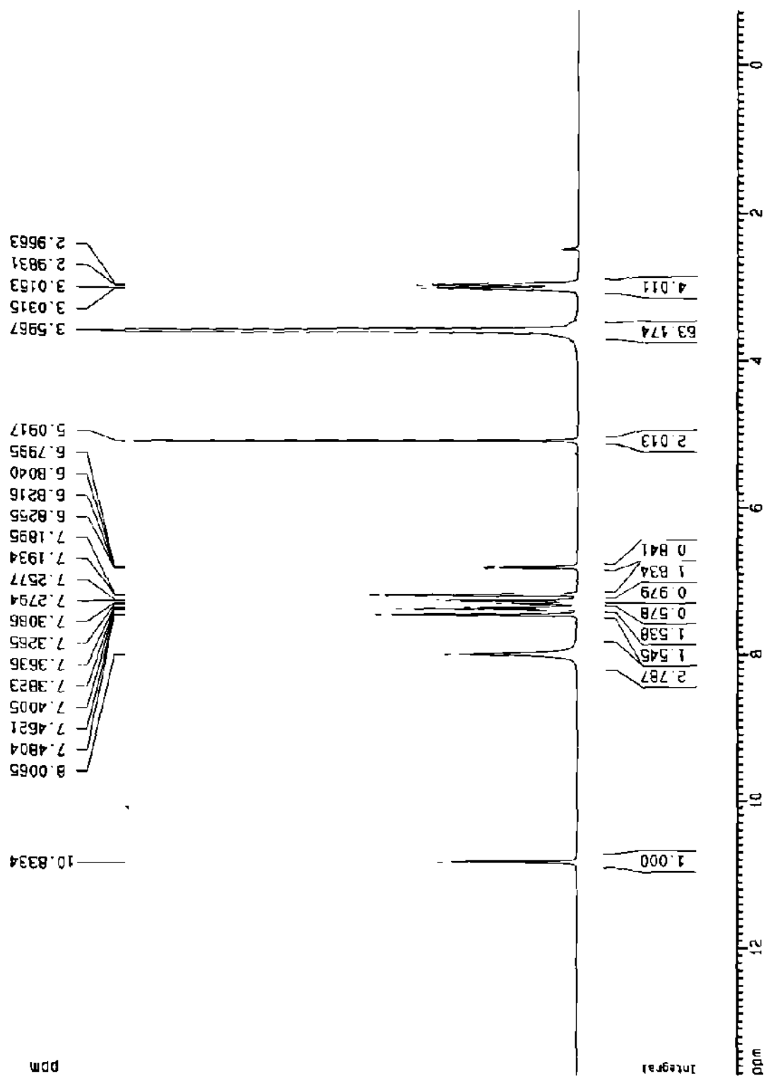
Fig. 10. Espectro de ^1\text{H} RMN del hidrocloreuro de 5-benciloxitriptamina
