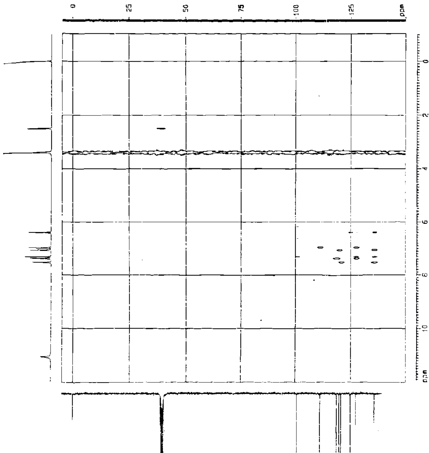
Fig. 31. Espectro de HMBC, del indol
