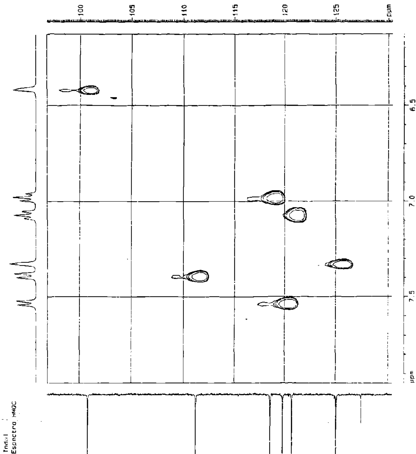
Fig. 26. Espectro de HMQC, del indol
