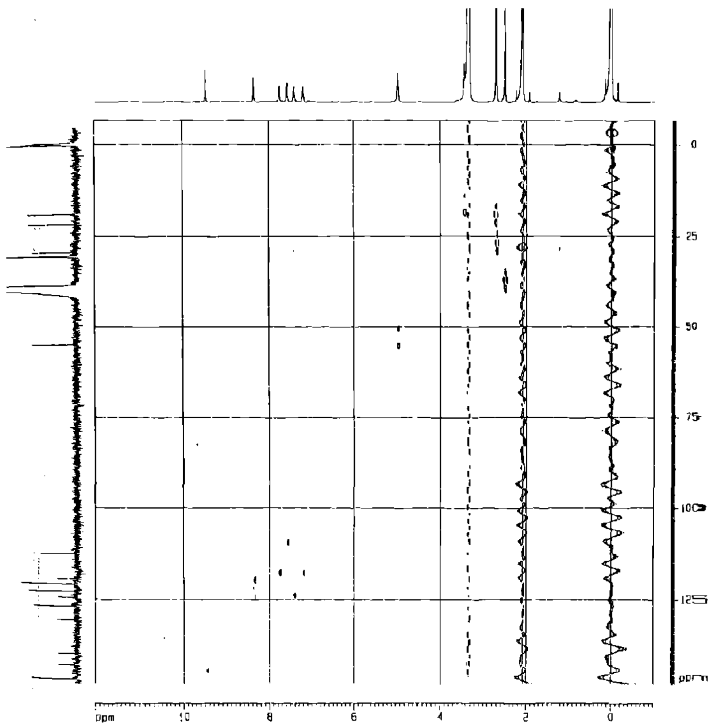
Fig. 52. Espectro de HMQC, de 24
