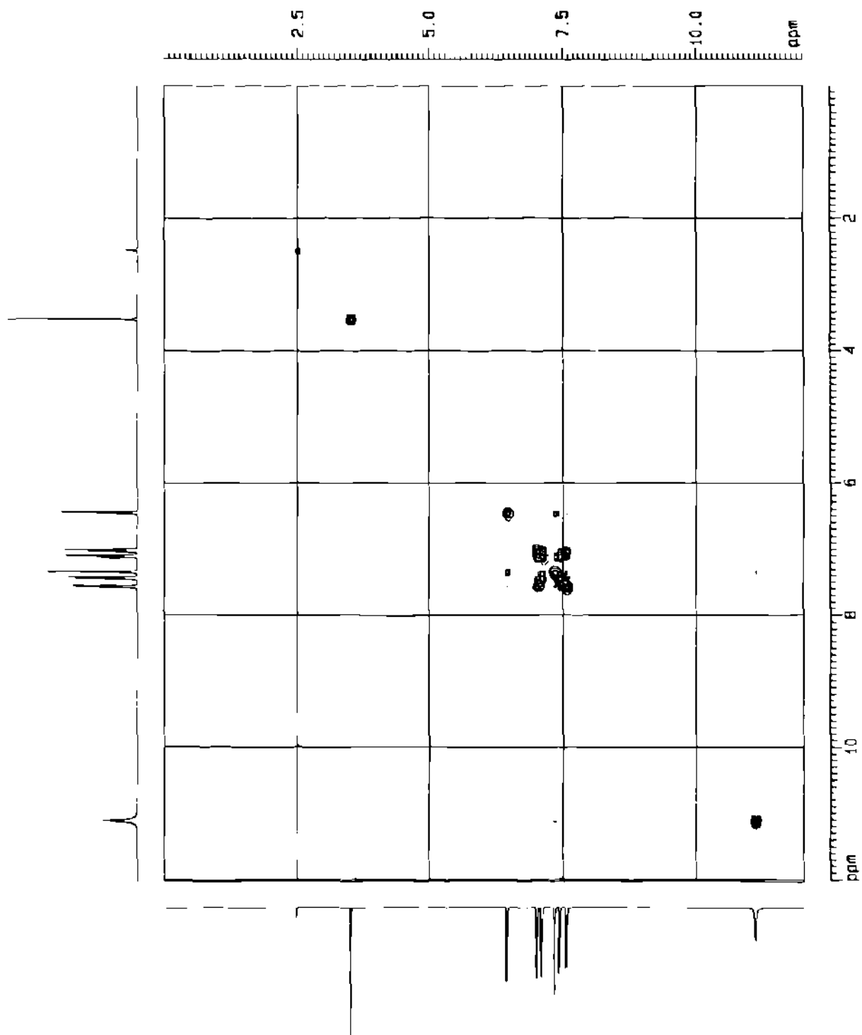
Fig. 11. Espectro de 2D ^1\text{H} RMN, Cosy del indol
