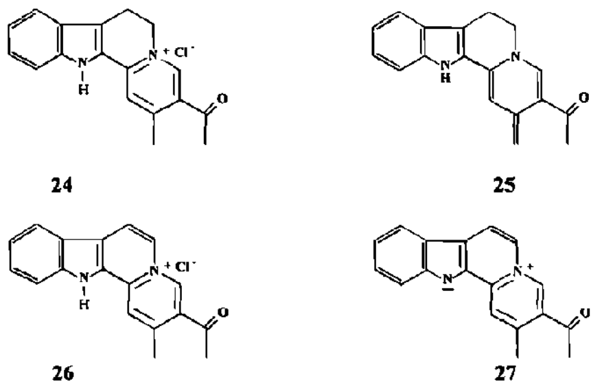
Fig. 4. Sustancias con la estructura base de indoloquinolizina sintetizadas por Teuber.
