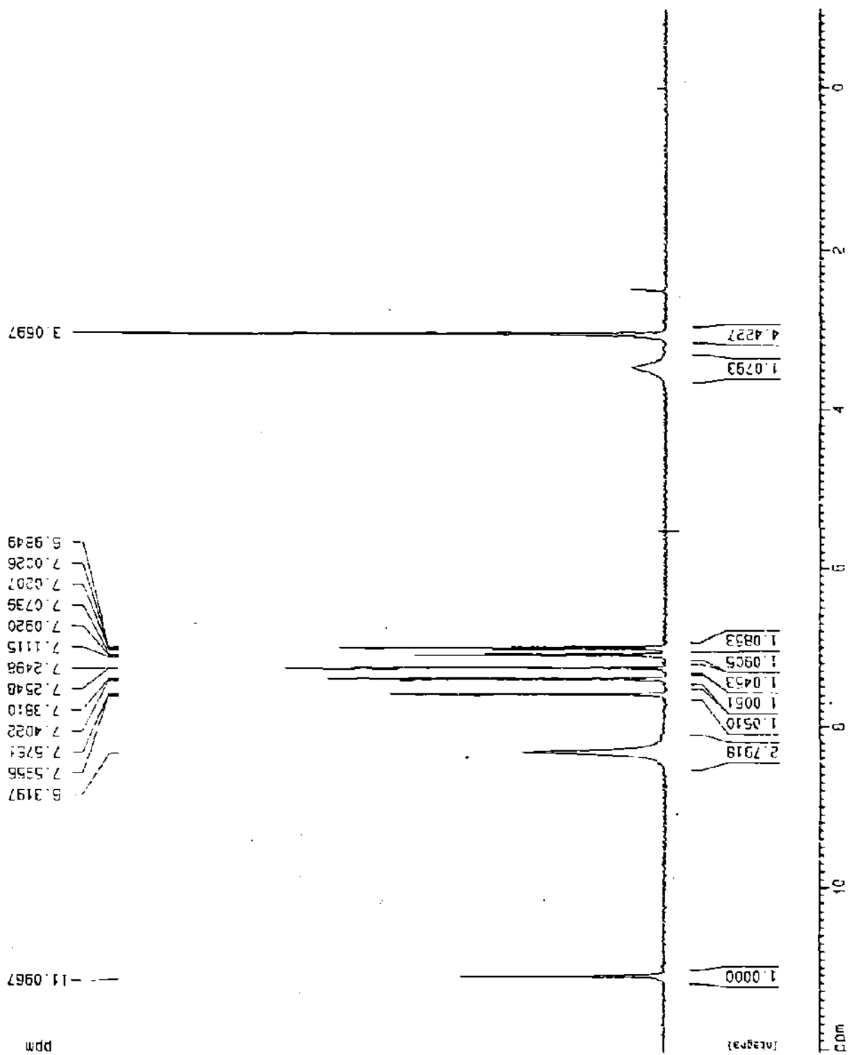
Fig. 8. Espectro de ^1\text{H} RMN del hidrocloreuro de triptamina
