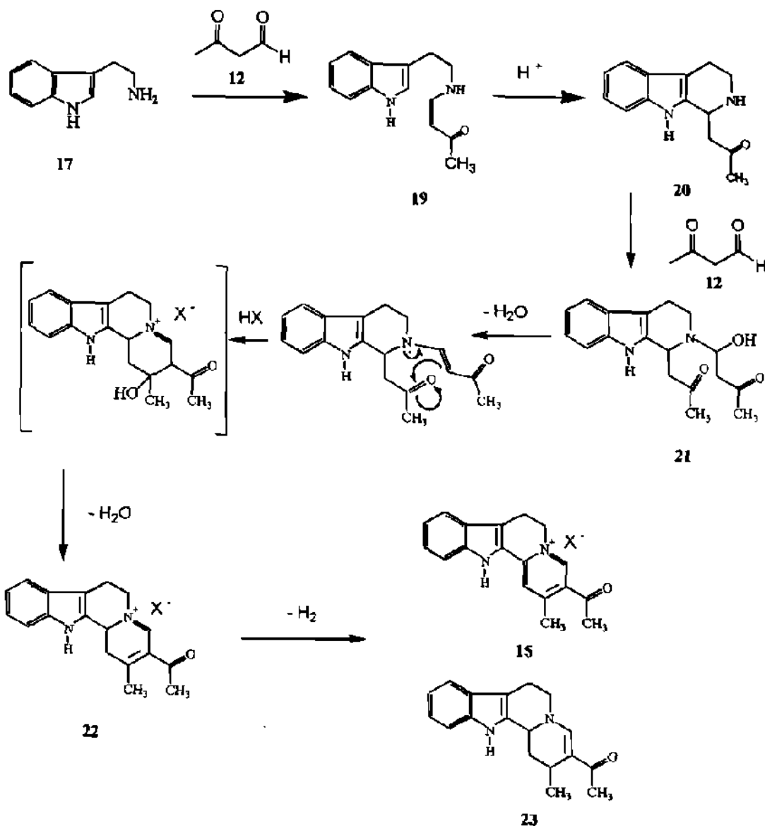
Fig. 3. Mecanismo propuesto de la reacción de Teuber
