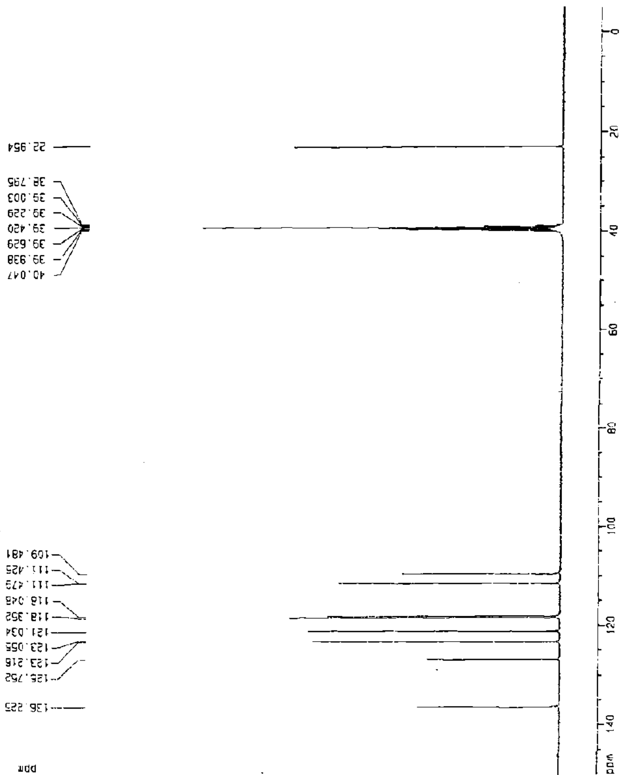
Fig. 18. Espectro de ^{13}\text{C} RMN, del hidrocloreuro de triptamina
