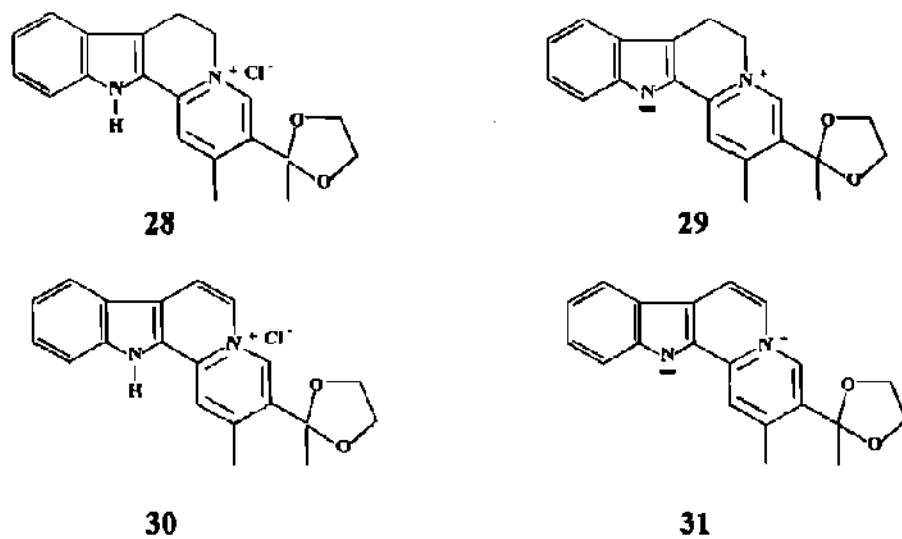
Fig. 5. Sustancias con la estructura base de indoloquinolizina sintetizadas por Quintanilla
