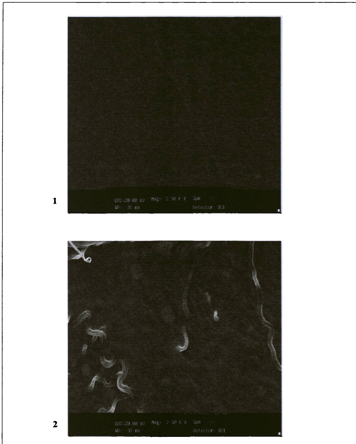
Fig.40. Micrografía electrónica de Barrido de la película 3 A 1 a las cero horas (1) y a las 192 horas (2).
