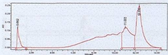
Tuberilina
