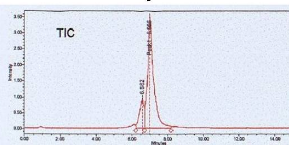
Baileyolona
