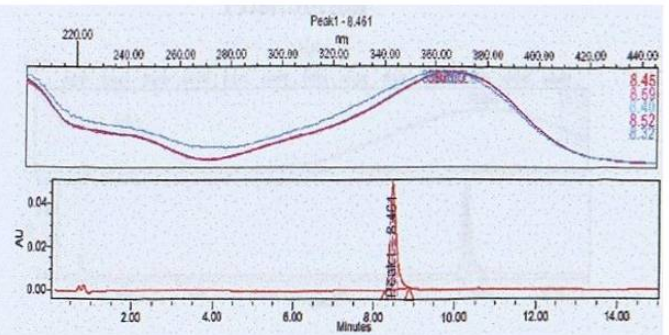
Kukulkanina A
