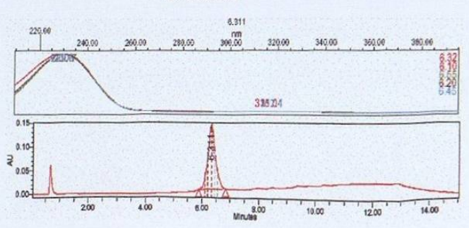
Tenulina
