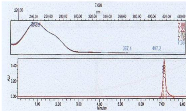
Santonina
