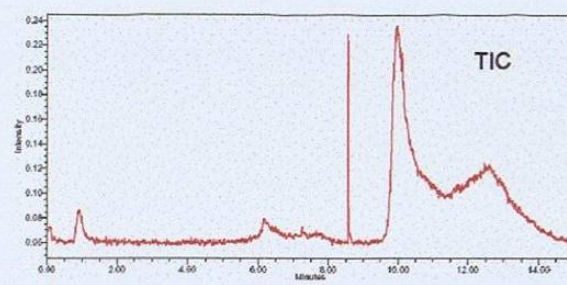
Quercitrina
