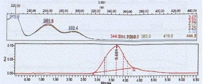
Ácido vainílico
