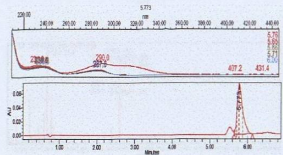
Criptopina
