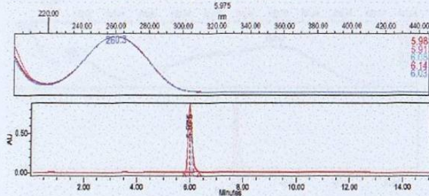
Kukulkanina B
