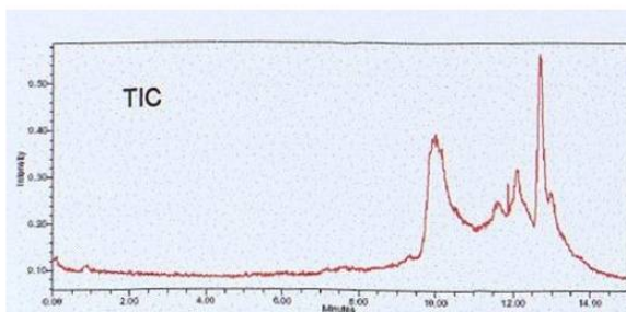
Acetato b-amirina
