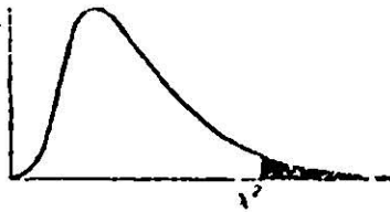
Cuadro 6. Distribuciones \chi^2
