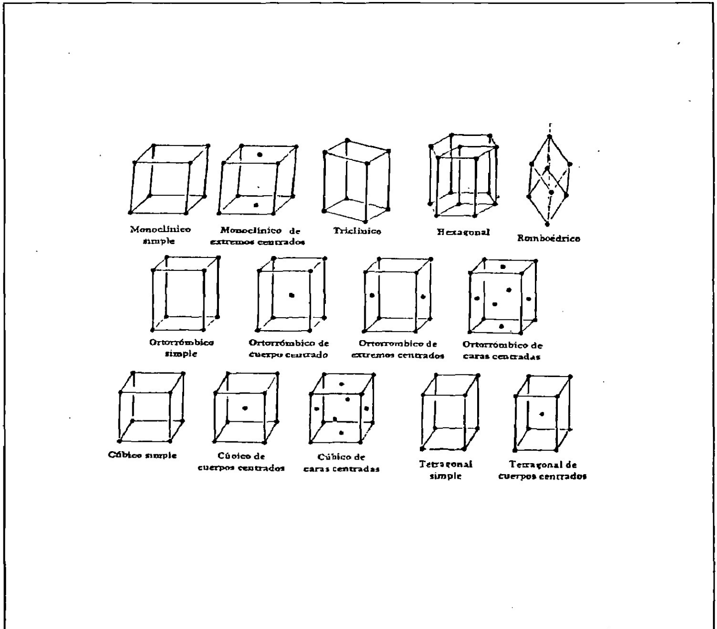
Los siete sistemas de estructura cristalina y las 14 redes de Bravais
