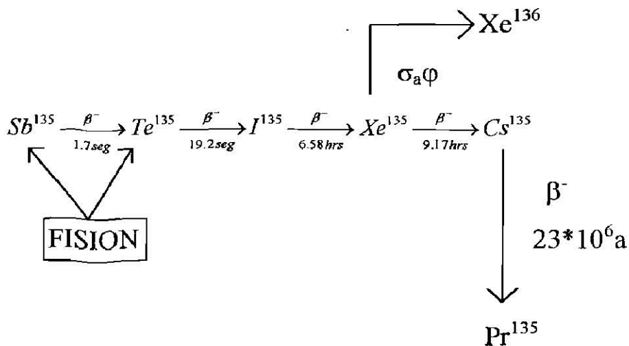
PRODUCCION DEL XENON-135
