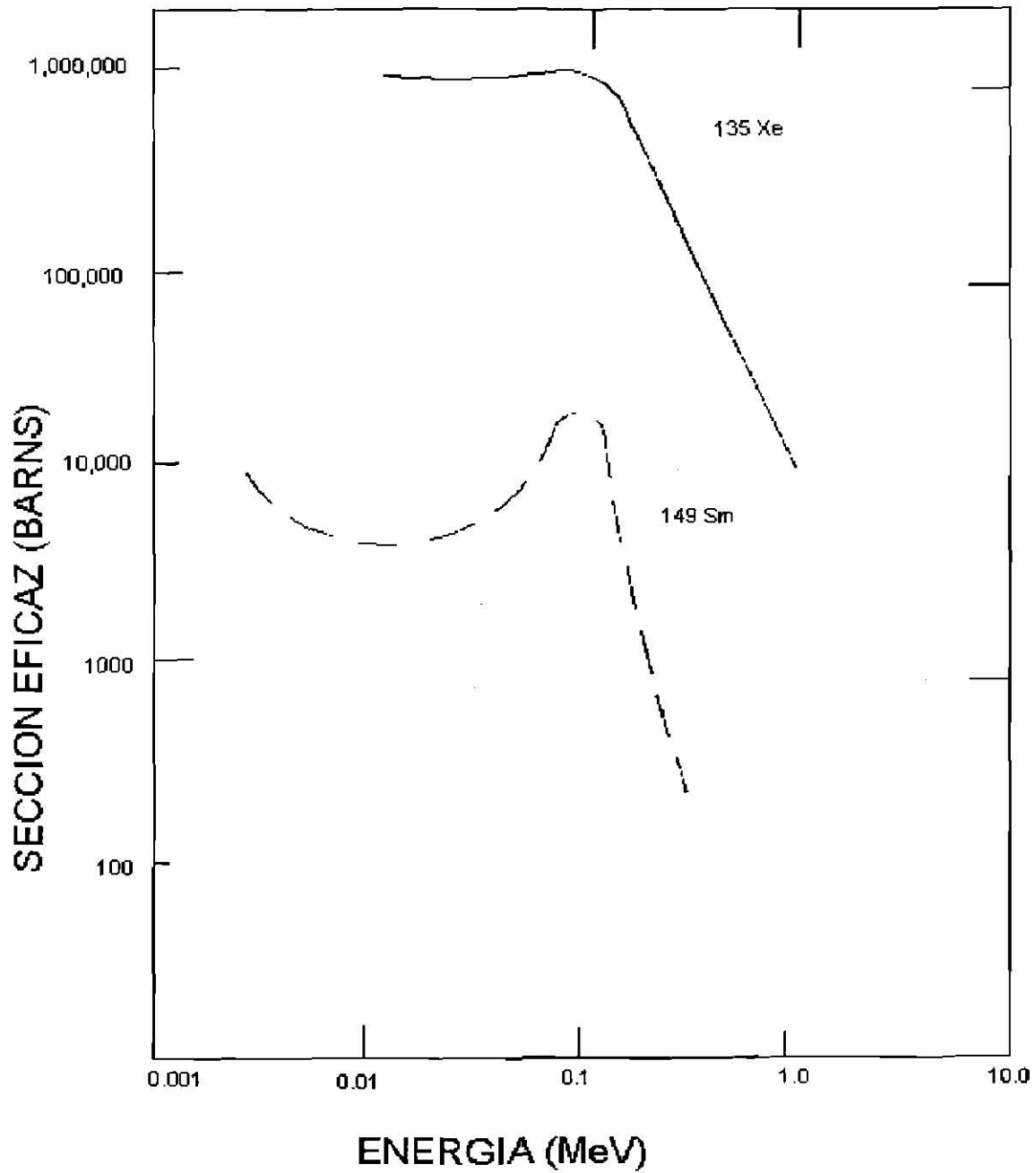
FIGURA 11 SECCIÓN EFICAZ DE XENON-135 Y DEL SAMARIO 149.
