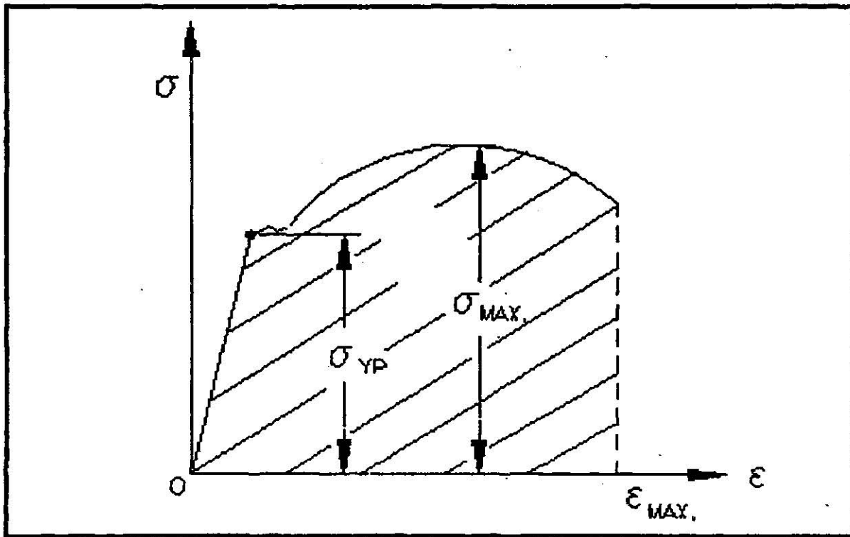
Figura 3.6a Obtención de la Tenacidad
