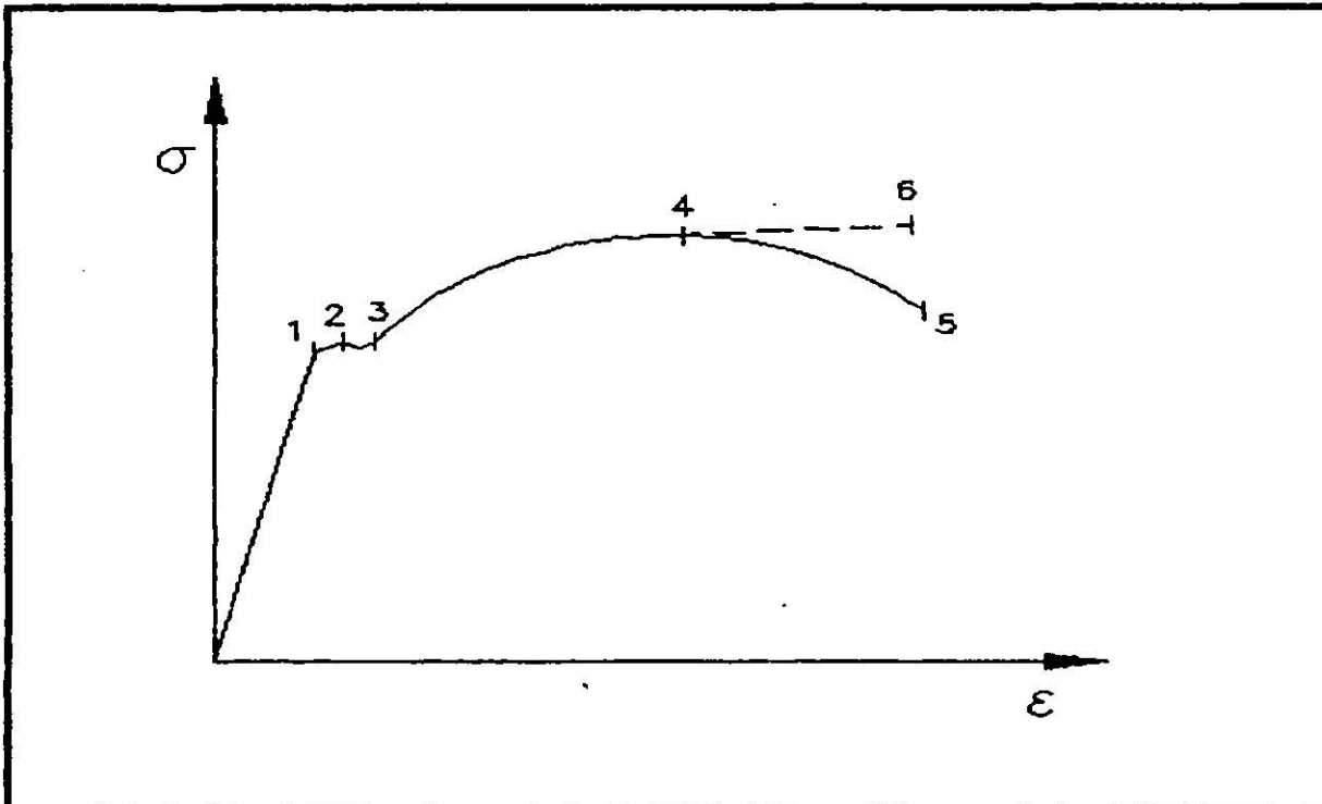
Figura 3.1 Gráfica Esfuerzo vs. Deformación unitaria
