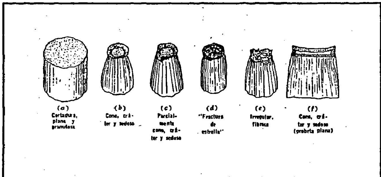
Figura 3.13 Fracturas típicas por tensión en metales.
