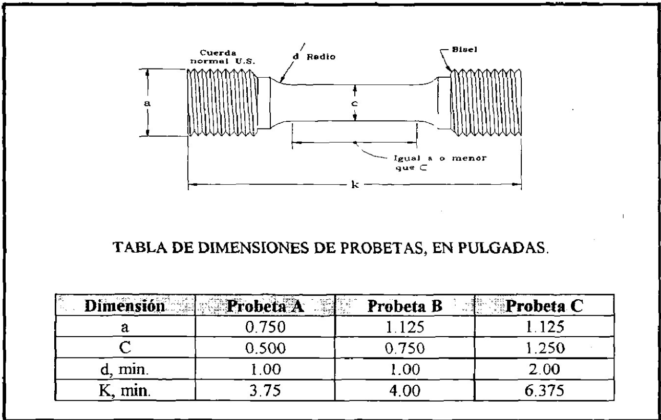
Figura 3.11 Estándar para Hierro fundido A.S.T.M. E-8, A 48
