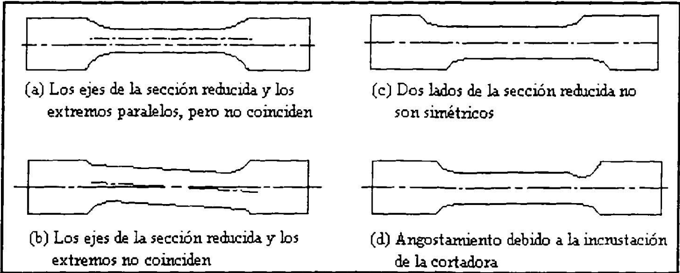
Figura 3.8 Defectos comunes en las probetas planas
