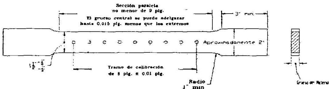
(c) Probeta rectangular estándar con tramo de calibración de 8 plg. para ensaye de metales en forma de placa, lámina, etc., con grueso de 3/16 plg. o más.
