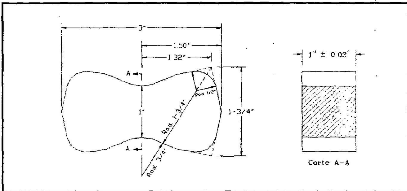
Figura 3.12 Estándar A.S.T.M. C150, C190, para concreto y cemento portland
