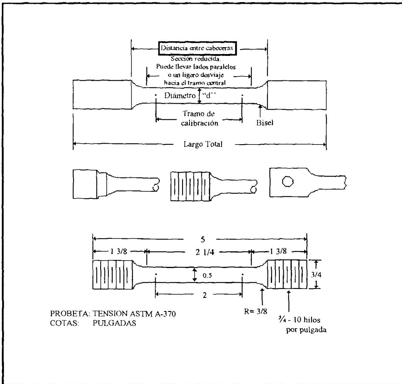
Figura 3.7 Tipos de extremos para probetas de tensión
