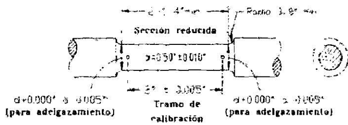
(a) Probeta redonda estándar con tramo de calibración de 2 plg.
