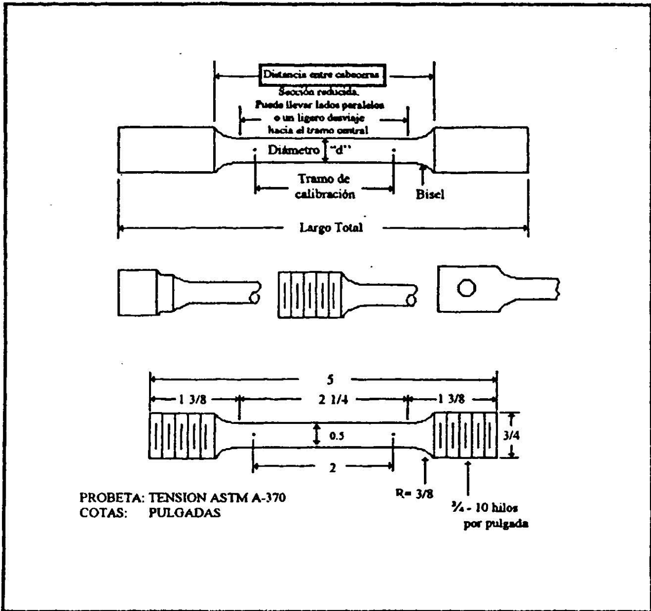
Figura 3.7 Tipos de extremos para probetas de tensión
