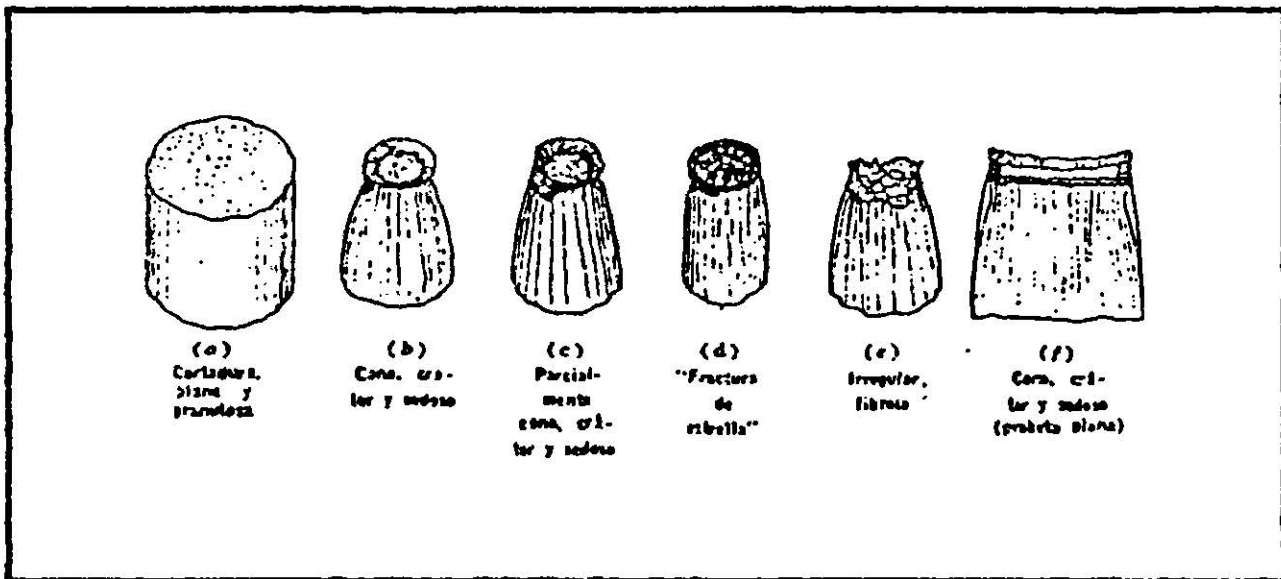
Figura 3.13 Fracturas típicas por tensión en metales.
