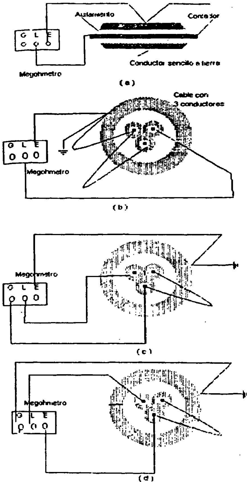
Figura 2.4 Conexiones de la prueba de cable para medición de la resistencia de aislamiento: (a) Conexión para la prueba de un conductor sencillo y un conductor a tierra. (b) Conexión para un cable de tres conductores, un conductor a otro conductor y el envoltorio a tierra. (c) Conexión para un cable de tres conductores, un conductor a la vaina y a tierra y dos conductores protegidos. (d) Conexión para un cable de tres, un conductor a todos los otros conductores sin pérdidas por tierra.
