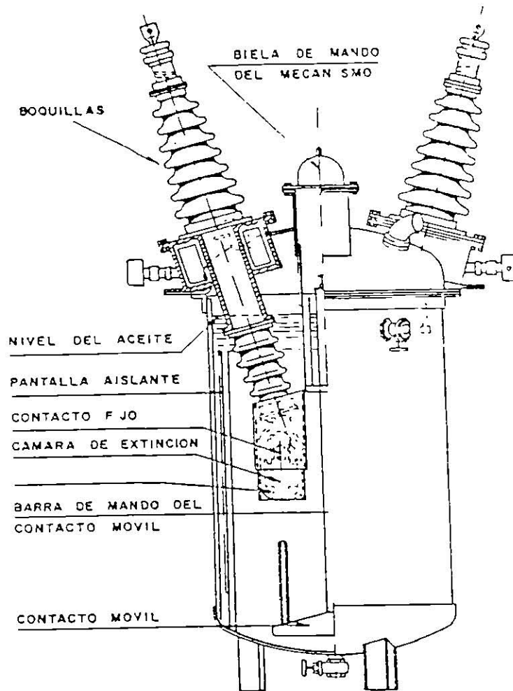
Figura 1.5. Interruptor de gran volumen de aceite.
