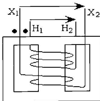
Figura 3.2. Polaridad aditiva.
