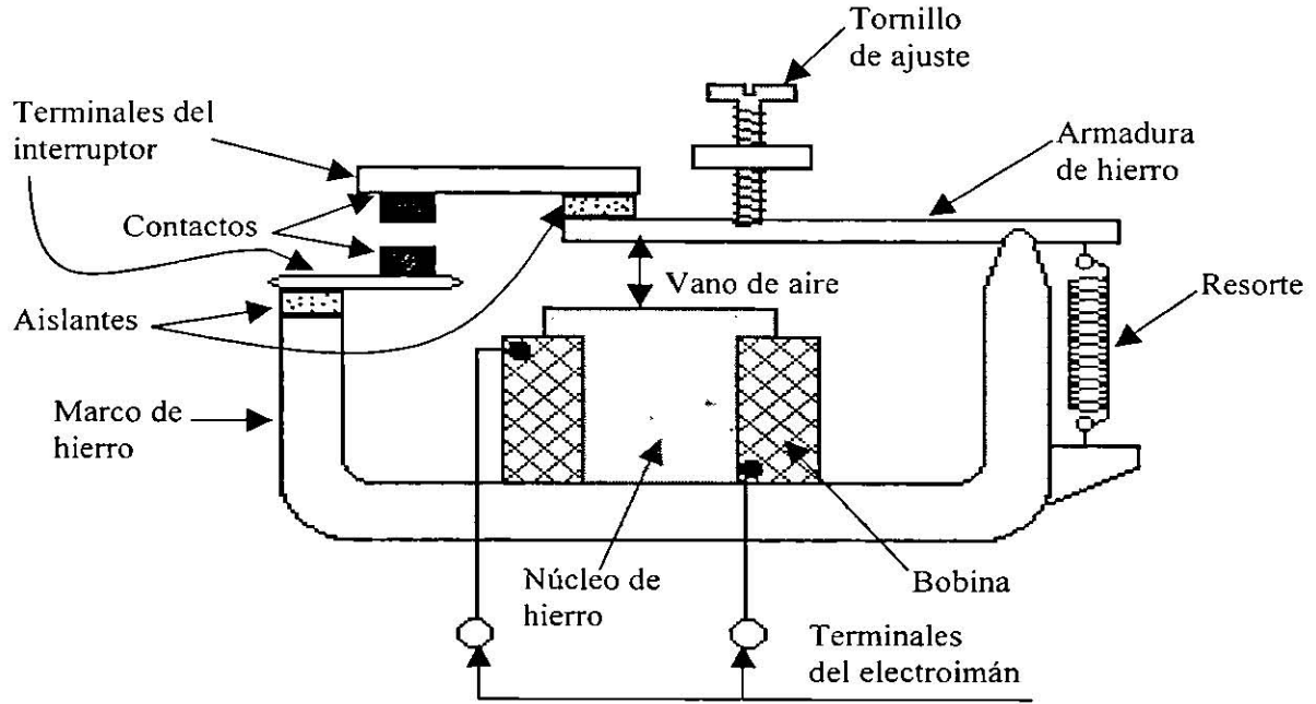
Figura 1.9. Relé tipo bisagra
