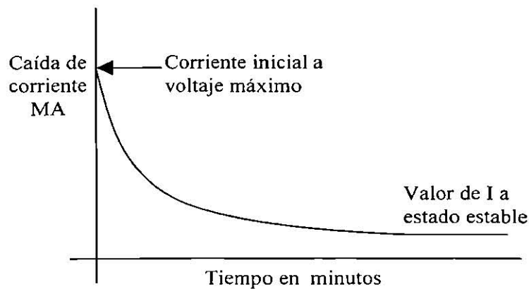
Figura 2.7. Caída de corriente contra tiempo.
