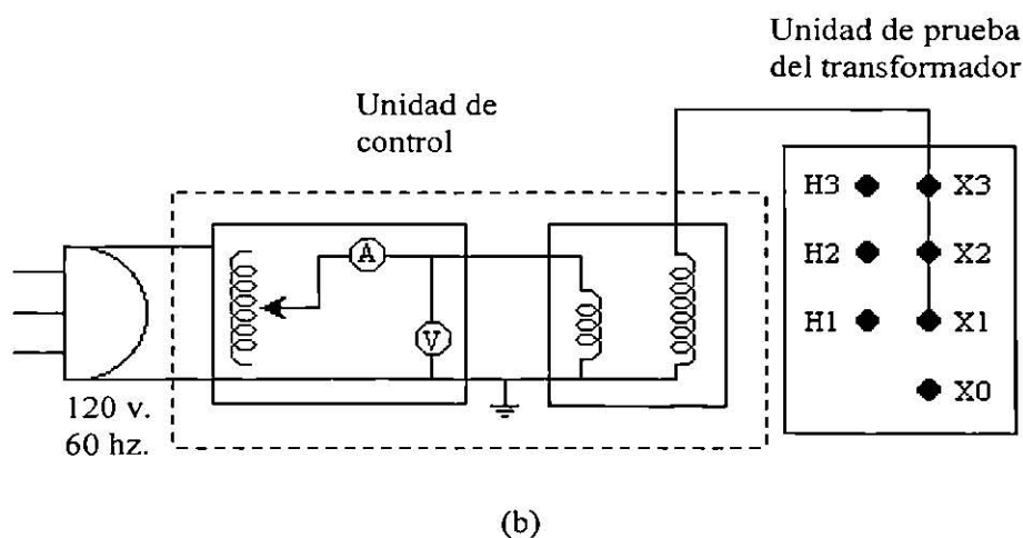
Figura 2.5. Conexión de la prueba de Hi-pot; (a) Conexión en las bobinas de alta; (b) Conexión de las bobinas de baja.
