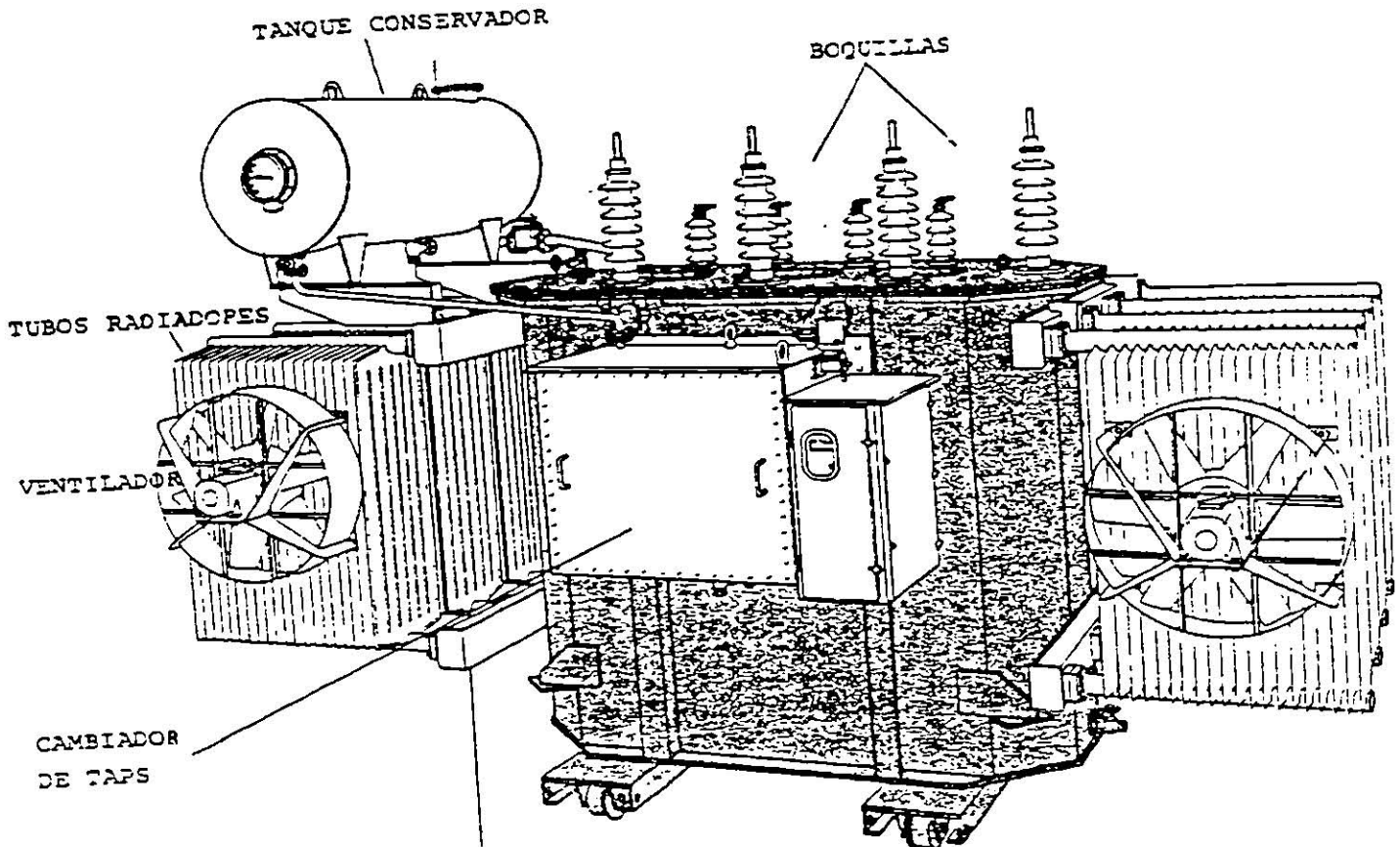
Figura 2.1. Transformador de potencia.
