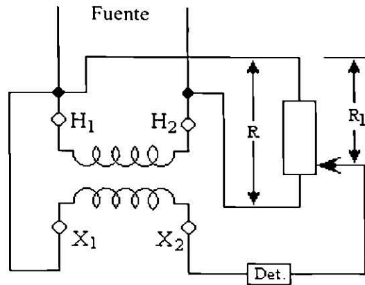
Figura 3.7. Potenciometro de resistencia para la prueba de razón
