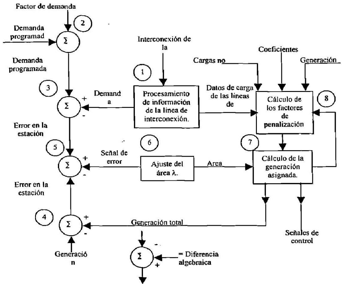
Figura 1.1. Diagrama de bloques.
