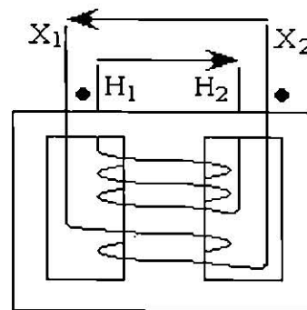
Figura 3.3. Polaridad sustractiva.
