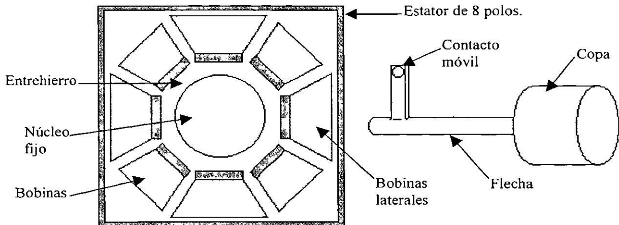
Figura 1.12. Relé de copa de inducción.
