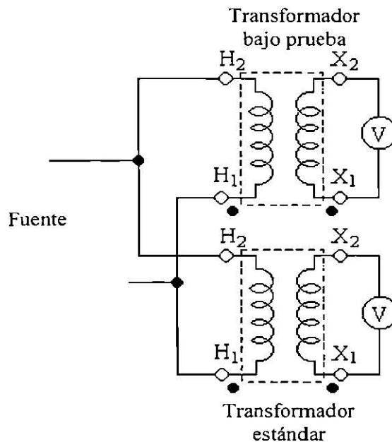
Figura 3.6. Voltímetro dispuesto para leer los voltajes de secundario, después de intercambiar.
