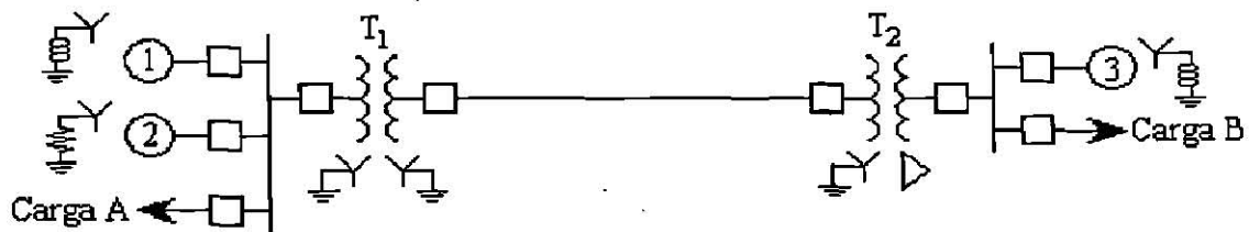
Figura 1.2. Diagrama unifilar.
