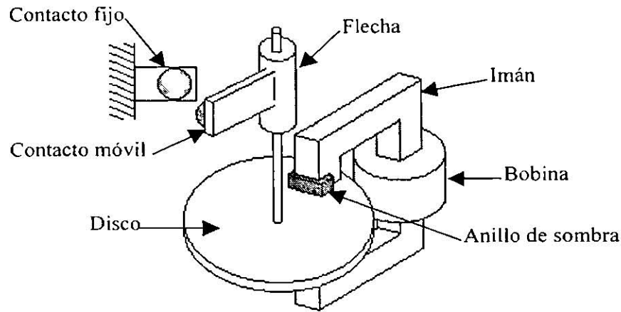
Figura 1.11. Relé de disco de inducción.
