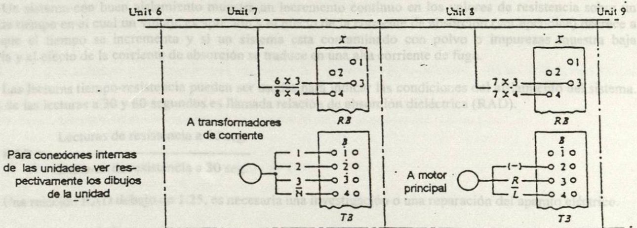
(c) Diagrama de interconexión
