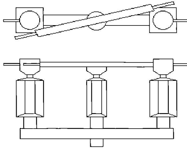
Figura 1.7 (a). Cuchilla desconectadora de tres columnas con accionamiento en la columna central .
