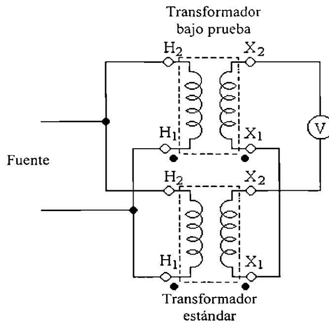
Figura 3.5. Voltímetro dispuesto para leer la diferencia entre los dos voltajes de secundario.
