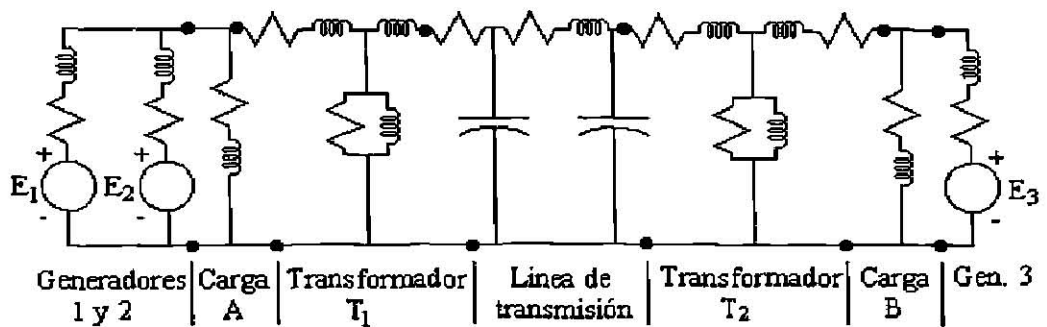
Figura 1.3. Diagrama de impedancias y reactivancias.
