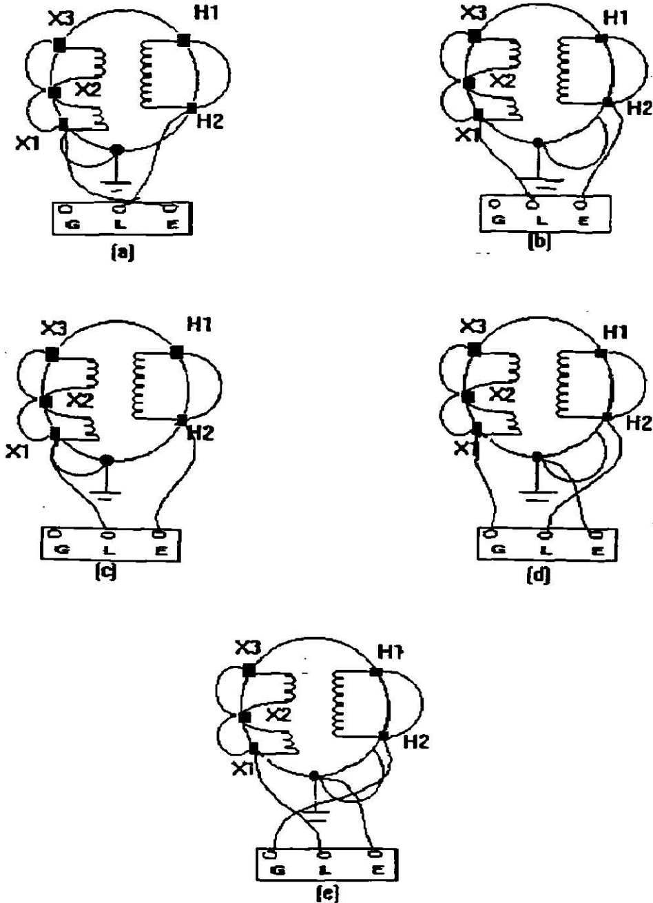
Fig. 2.1 Prueba de conexiones para aislamiento resistivo de transformadores de una sola fase
