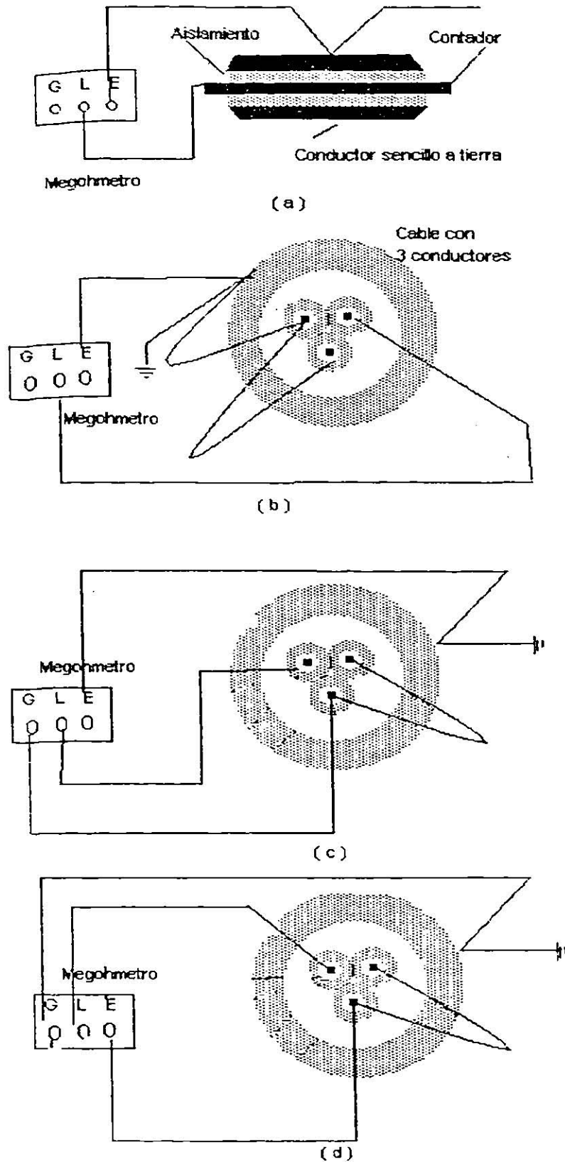
Figura 2.4 Conexiones de la prueba de cable para medición de la resistencia de aislamiento: (a) Conexión para la prueba de un conductor sencillo y un conductor a tierra. (b) Conexión para un cable de tres conductores, un conductor a otro conductor y el envolvente a tierra. (c) Conexión para un cable de tres conductores, un conductor a la vaina y a tierra y dos conductores protegidos. (d) Conexión para un cable de tres, un conductor a todos los otros conductores sin pérdidas por tierra.
