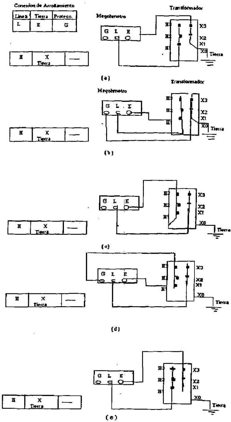
Fig. 2.2 Conexiones de prueba para resistencia de aislamiento para transformadores trifasicos. ( a ) Conexiones de bobina de alta a bobina de baja a tierra; ( b ) Conexión para bobina de alta a tierra y bobina de alta protegida; ( c ) Conexión de bobina de baja a bobina de alta a tierra; ( d ) Conexión de bobina de bobina de baja a tierra y bobina de alta y protegida; ( e ) Conexión de bobina de alta a bobina de baja.
