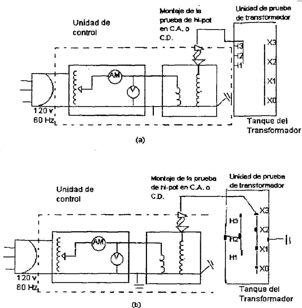
Fig. 2.3 Conexión de la prueba de alto voltaje del transformador ( HI - POT ). (a) Conexión de la prueba HI - POT en las bobinas de alta. (b) Conexión de la alta de la prueba de HI - POT en las bobinas de baja.
