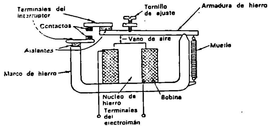
Fig. 1.7(a) Relé básico
