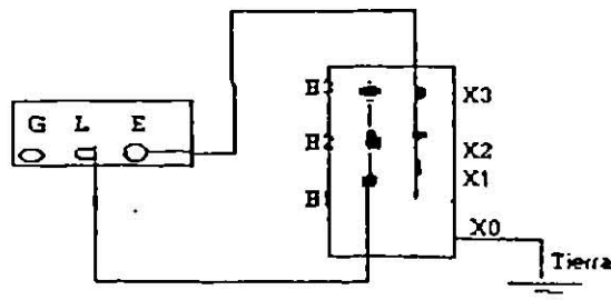
Fig. 2.2 Conexiones de prueba para resistencia de aislamiento para transformadores trifasicos. ( a ) Conexiones de bobina de alta a bobina de baja a tierra; ( b ) Conexión para bobina de alta a tierra y bobina de alta protegida; ( c ) Conexión de bobina de baja a bobina de alta a tierra; ( d ) Conexión de bobina de bobina de baja a tierra y bobina de alta y protegida; ( e ) Conexión de bobina de alta a bobina de baja.
