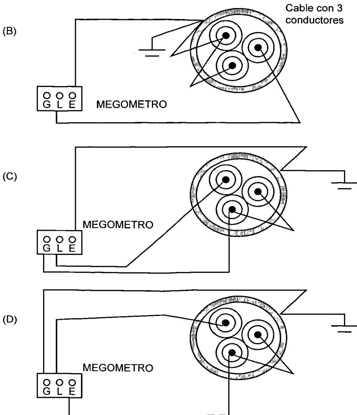
Figura 2.4 Conexiones de la prueba de cable para medición de la resistencia del aislamiento.
