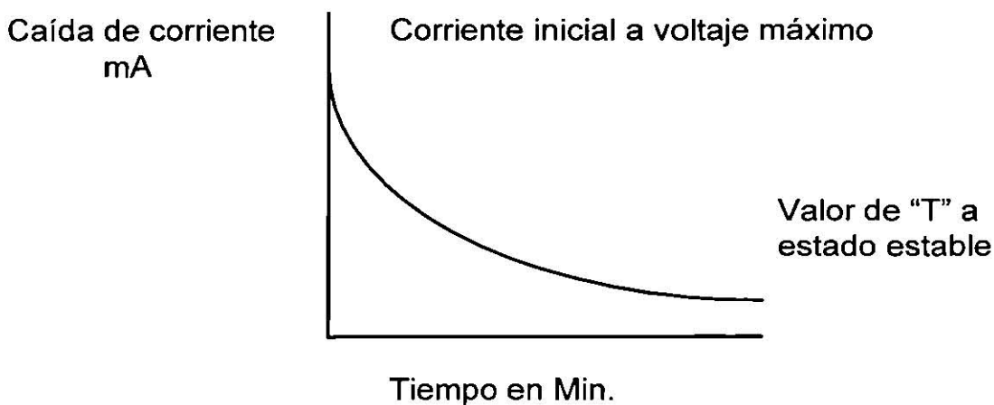
Figura 2.7 Caída de corriente contra tiempo.
