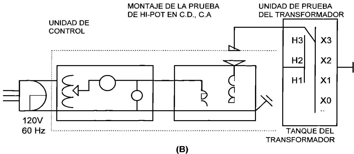
FIGURA 2.3 Conexión de la prueba de alto voltaje del transformador (HI-POT): A) Conexión de la prueba HI-POT en las bobinas de alta. B) Conexión de la prueba HI-POT en las bobinas de baja.
