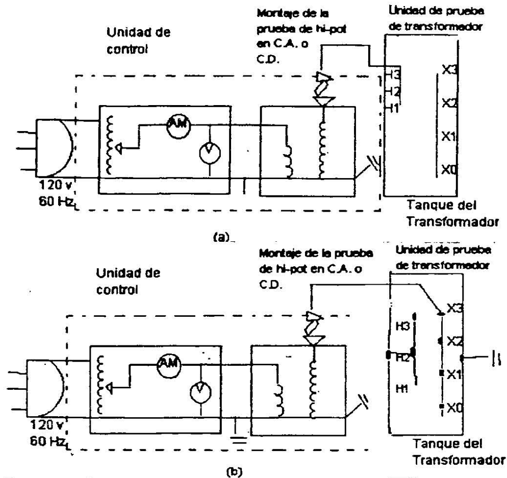
Fig. 2.3 Conexión de la prueba de alto voltaje del transformador ( HI - POT ). (a) Conexión de la prueba HI - POT en las bobinas de alta. (b) Conexión de la alta de la prueba de HI - POT en las bobinas de baja.
